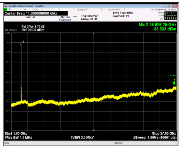
38-38-20MHz-20MHz-QPSK-QPSK-37850-38048-1RB#0-1 RB#99-1000~27000MHz-PASS
