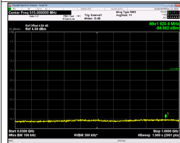
41(2555-2655)-41(2555-2655)-5MHz-20MHz-16QAM-16 QAM-40273-40390-1RB#0-1RB#99-30~1000MHz-PASS
