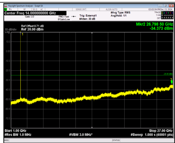
41(2555-2655)-41(2555-2655)-5MHz-20MHz-16QAM-16QA M-40273-40390-1RB#0-0RB#0-1000~27000MHz-PASS
