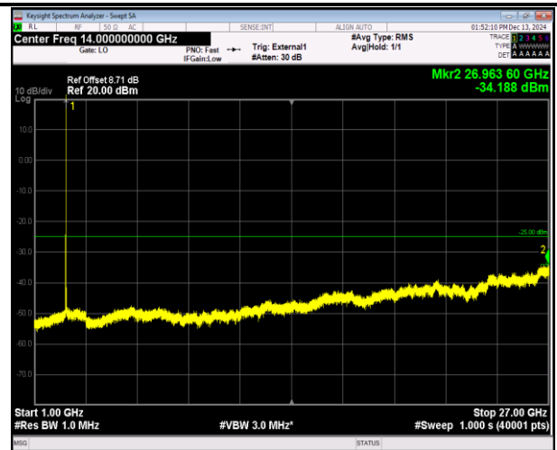
38-38-20MHz-20MHz-QPSK-QPSK-37952-38150-1RB#99- ORB#0-1000~27000MHz-PASS
