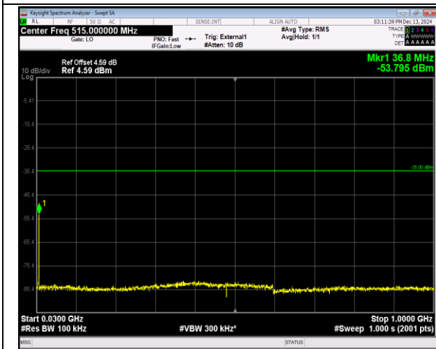
41(2555-2655)-41(2555-2655)-5MHz-20MHz-QPSK-QPS K-40648-40765-1RB#24-0RB#0-30~1000MHz-PASS
