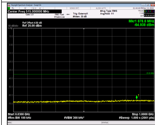
38-38-20MHz-20MHz-QPSK-QPSK-37901-38099-1RB#99-9-ORB#0-30~1000MHz-PASS
