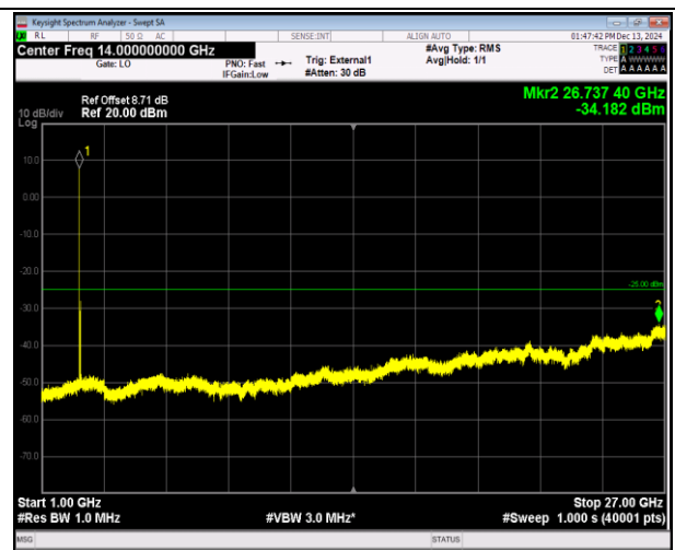
38-38-20MHz-20MHz-16QAM-16QAM-37901-38099-1RB# 0-1RB#99-1000~27000MHz-PASS
