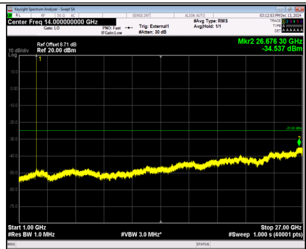
41(2555-2655)-41(2555-2655)-5MHz-20MHz-QPSK-QPSK- 40648-40765-1RB#24-0RB#0-1000~27000MHz-PASS
