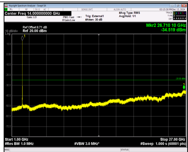
41(2555-2655)-41(2555-2655)-5MHz-20MHz-QPSK-QPSK- 40648-40765-25RB#0-100RB#0-1000~27000MHz-PASS
