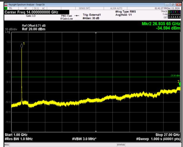
38-38-20MHz-20MHz-QPSK-QPSK-37850-38048-100RB#0 -100RB#0-1000~27000MHz-PASS
