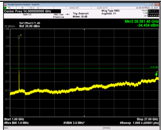
38-38-20MHz-20MHz-QPSK-QPSK-37901-38099-1RB#0-1RB#99-1000~27000MHz-PASS
