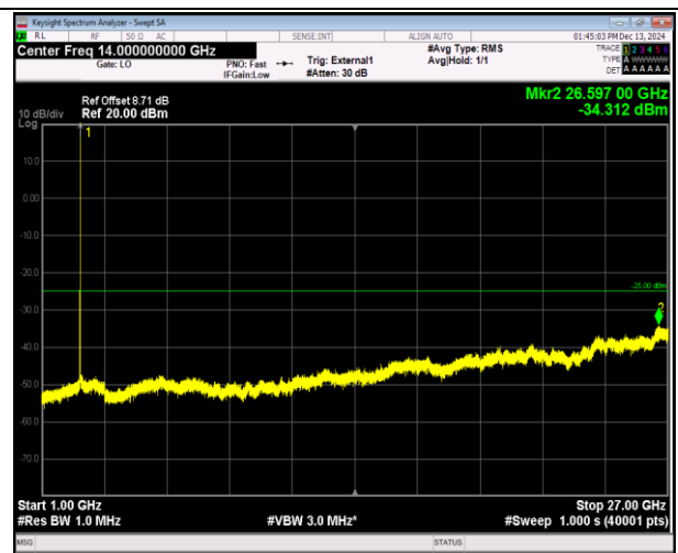
38-38-20MHz-20MHz-QPSK-QPSK-37901-38099-1RB#99-9-ORB#0-1000~27000MHz-PASS
