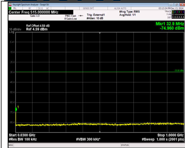
41(2555-2655)-41(2555-2655)-5MHz-20MHz-QPSK-QPS K-40648-40765-1RB#0-1RB#99-30~1000MHz-PASS
