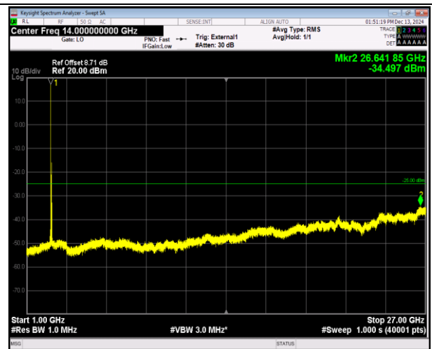
38-38-20MHz-20MHz-16QAM-16QAM-37952-38150-1RB# 0-ORB#0-1000~27000MHz-PASS
