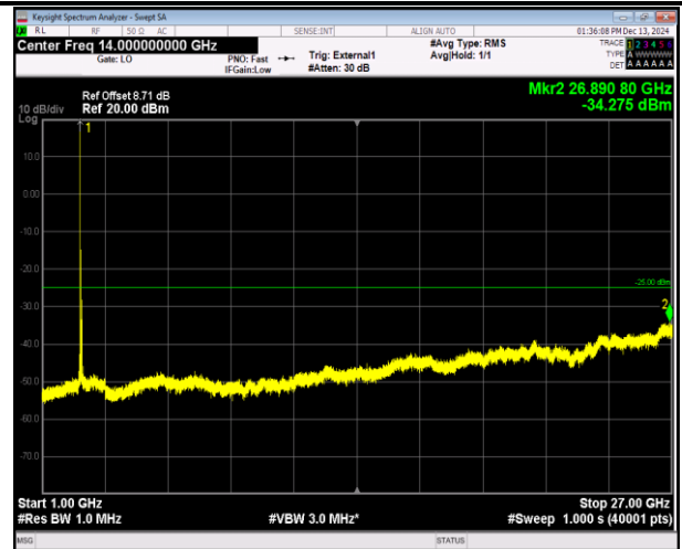
38-38-20MHz-20MHz-QPSK-QPSK-37850-38048-1RB#0-0 RB#0-1000~27000MHz-PASS
