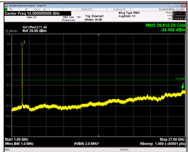
38-38-20MHz-20MHz-QPSK-QPSK-37901-38099-100RB#0-100RB#0-1000~27000MHz-PASS
