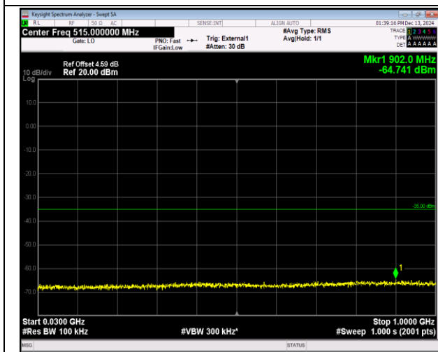
38-38-20MHz-20MHz-QPSK-QPSK-37850-38048-1RB#0- 1RB#99-30~1000MHz-PASS
