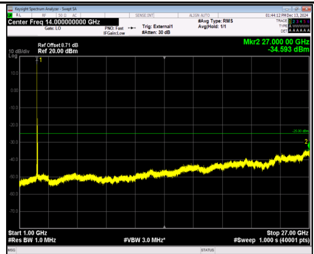
38-38-20MHz-20MHz-16QAM-16QAM-37901-38099-1RB# 0-ORB#0-1000~27000MHz-PASS
