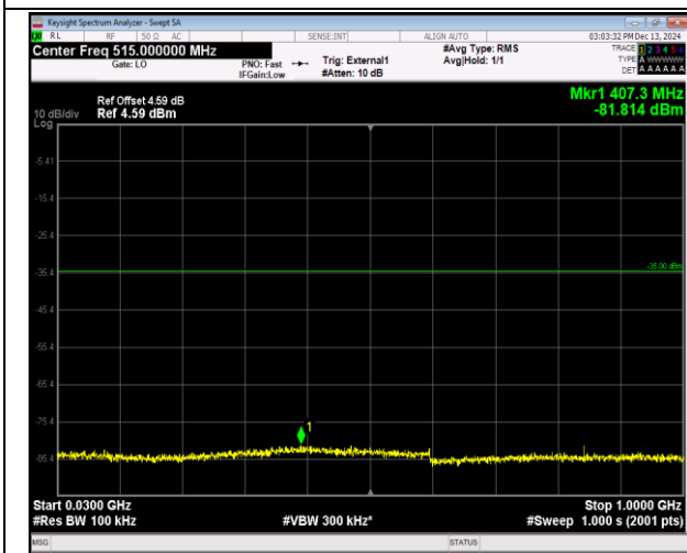
41(2555-2655)-41(2555-2655)-5MHz-20MHz-16QAM-16 QAM-40273-40390-1RB#0-0RB#0-30~1000MHz-PASS
