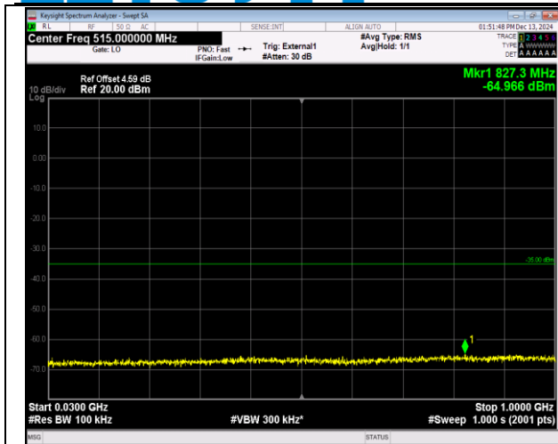
38-38-20MHz-20MHz-QPSK-QPSK-37952-38150-1RB#9 9-ORB#0-30~1000MHz-PASS
