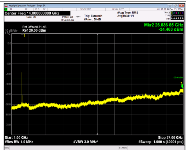
38-38-20MHz-20MHz-QPSK-QPSK-37850-38048-1RB#99- ORB#0-1000~27000MHz-PASS
