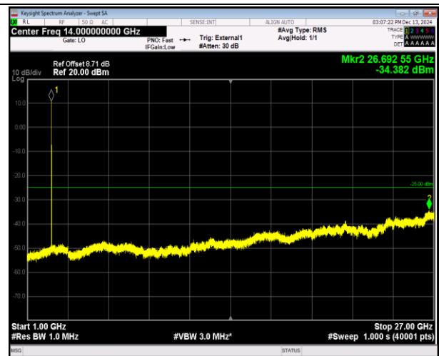
41(2555-2655)-41(2555-2655)-5MHz-20MHz-16QAM-16QA M-40273-40390-1RB#0-1RB#99-1000~27000MHz-PASS
