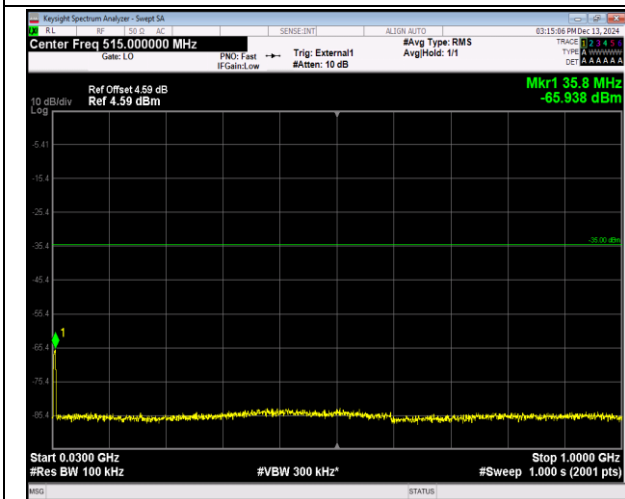
41(2555-2655)-41(2555-2655)-5MHz-20MHz-QPSK-QPS K-40648-40765-25RB#0-100RB#0-30~1000MHz-PASS
