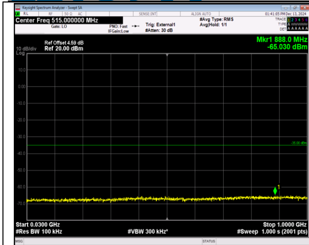
38-38-20MHz-20MHz-QPSK-QPSK-37850-38048-100RB #0-100RB#0-30~1000MHz-PASS
