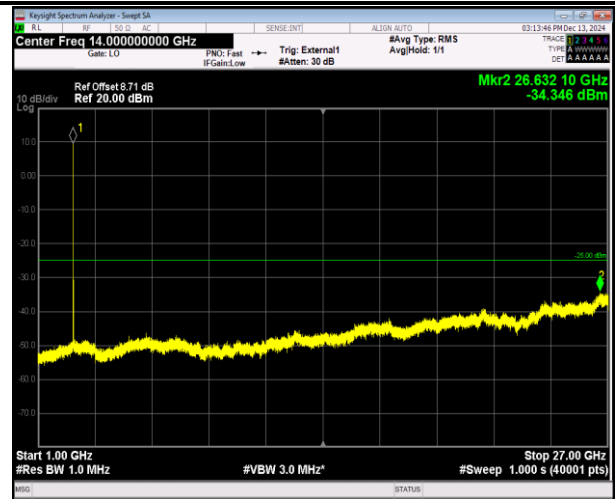
41(2555-2655)-41(2555-2655)-5MHz-20MHz-QPSK-QPSK- 40648-40765-1RB#0-1RB#99-1000~27000MHz-PASS
