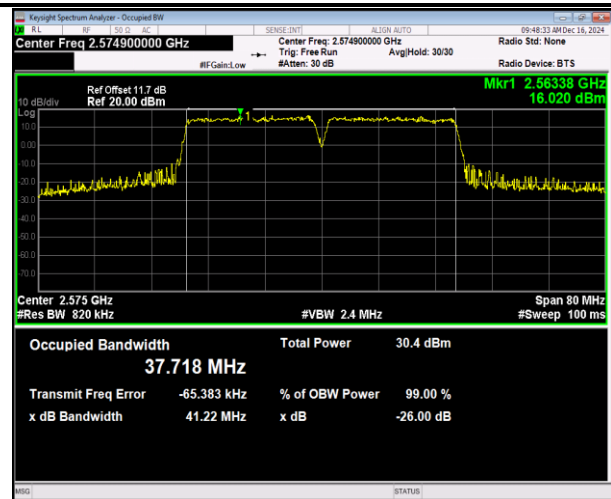
41(2555-2655)-41(2555-2655)-20MHz-20MHz-16QAM-16Q AM-40340-40538-100RB#0-100RB#0-PASS
