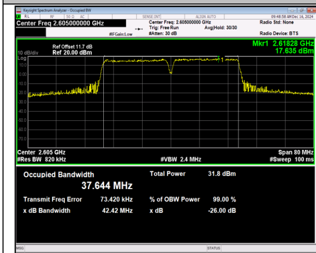
41(2555-2655)-41(2555-2655)-20MHz-20MHz-QPSK-QP SK-40641-40839-100RB#0-100RB#0-PASS
