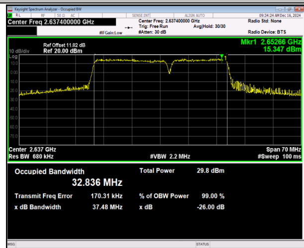
41(2555-2655)-41(2555-2655)-20MHz-15MHz-16QAM-16Q AM-40991-41162-100RB#0-75RB#0-PASS
