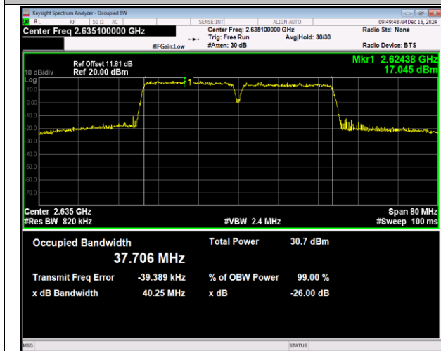
41(2555-2655)-41(2555-2655)-20MHz-20MHz-QPSK-QP SK-40942-41140-100RB#0-100RB#0-PASS
