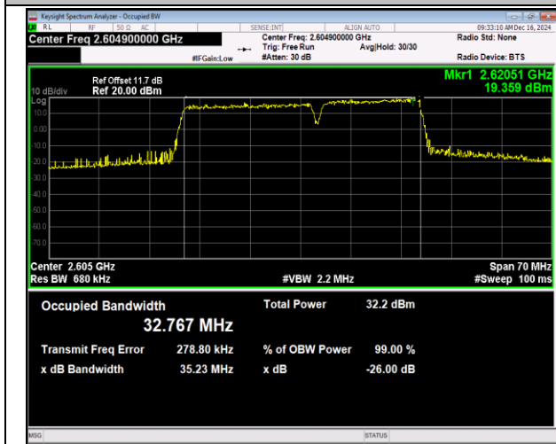
41(2555-2655)-41(2555-2655)-20MHz-15MHz-QPSK-QP SK-40666-40837-100RB#0-75RB#0-PASS
