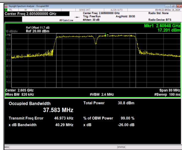
41(2555-2655)-41(2555-2655)-20MHz-20MHz-16QAM-16Q AM-40641-40839-100RB#0-100RB#0-PASS
