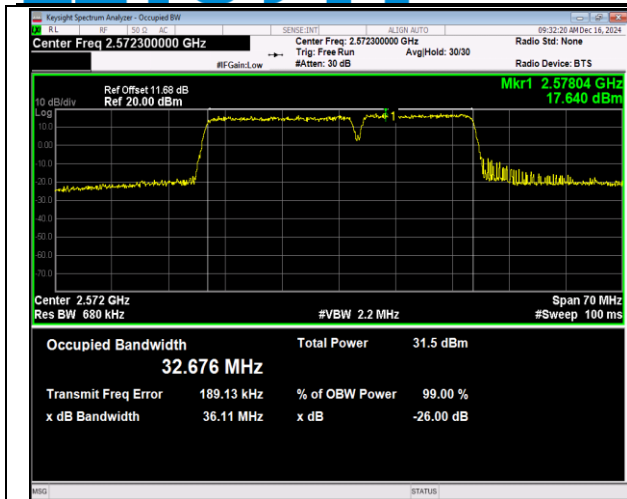
41(2555-2655)-41(2555-2655)-20MHz-15MHz-QPSK-QP SK-40340-40511-100RB#0-75RB#0-PASS
