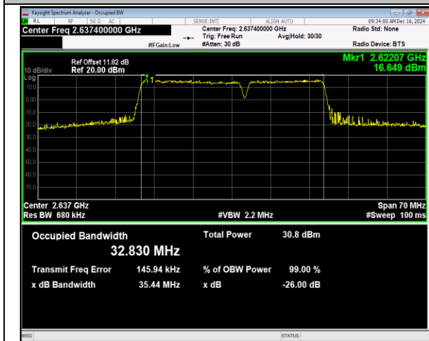
41(2555-2655)-41(2555-2655)-20MHz-15MHz-QPSK-QP SK-40991-41162-100RB#0-75RB#0-PASS
