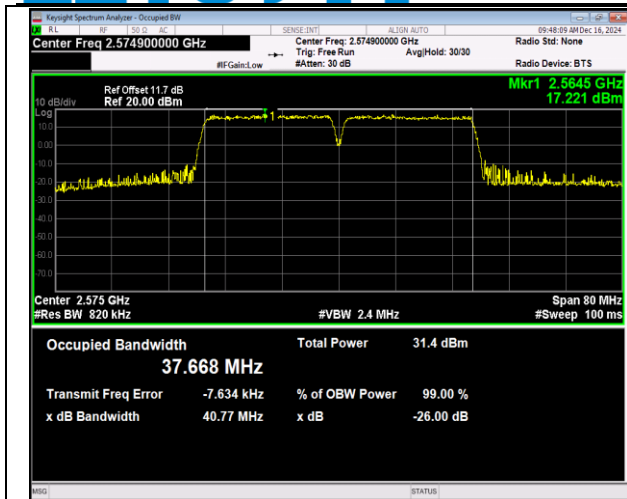
41(2555-2655)-41(2555-2655)-20MHz-20MHz-QPSK-QP SK-40340-40538-100RB#0-100RB#0-PASS
