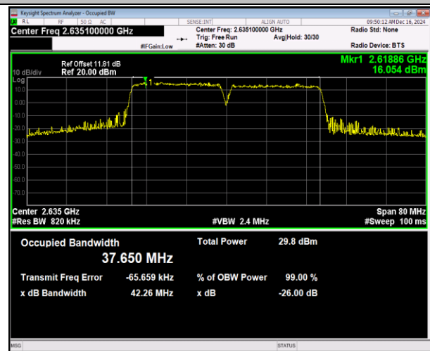
41(2555-2655)-41(2555-2655)-20MHz-20MHz-16QAM-16Q AM-40942-41140-100RB#0-100RB#0-PASS
