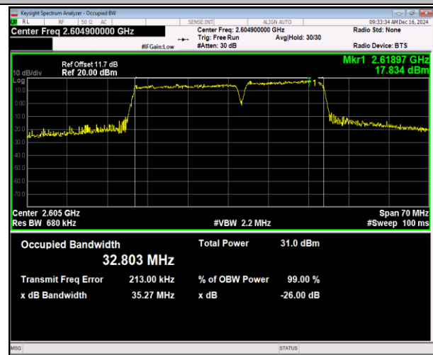
41(2555-2655)-41(2555-2655)-20MHz-15MHz-16QAM-16Q AM-40666-40837-100RB#0-75RB#0-PASS
