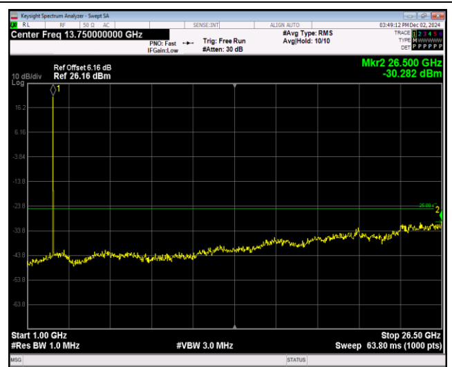
Band41-5MHz-QPSK-41215-1RB#0-Range2:1000~2 6500MHz
