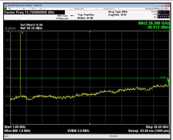
Band38-20MHz-QPSK-38150-1RB#0-Range2:1000~26500MHz
