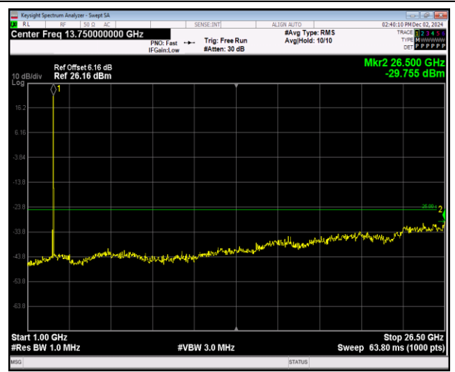
Band38-5MHz-QPSK-38000-1RB#0-Range2:1000~2 6500MHz
