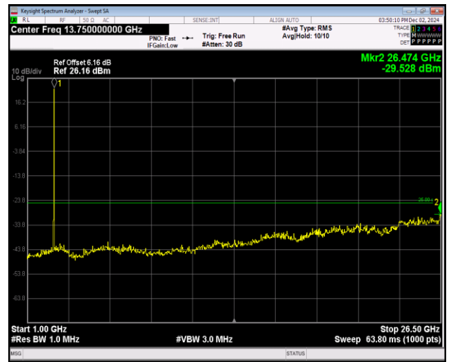
Band41-5MHz-16QAM-40065-1RB#0-Range2:1000~ 26500MHz
