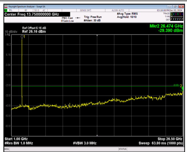
Band38-20MHz-QPSK-38000-1RB#0-Range2:1000~26500MHz
