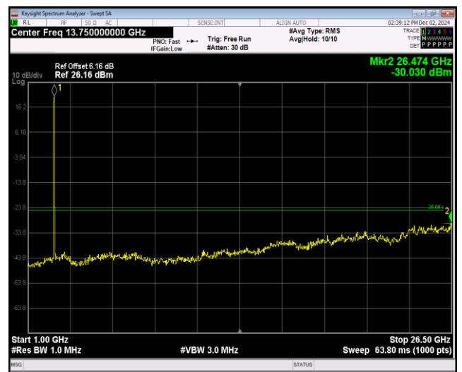
Band38-5MHz-QPSK-38000-1RB#0-Range2:1000~2 6500MHz
