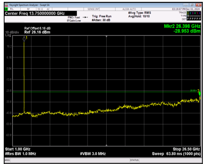
Band38-20MHz-QPSK-38150-1RB#0-Range2:1000~26500MHz
