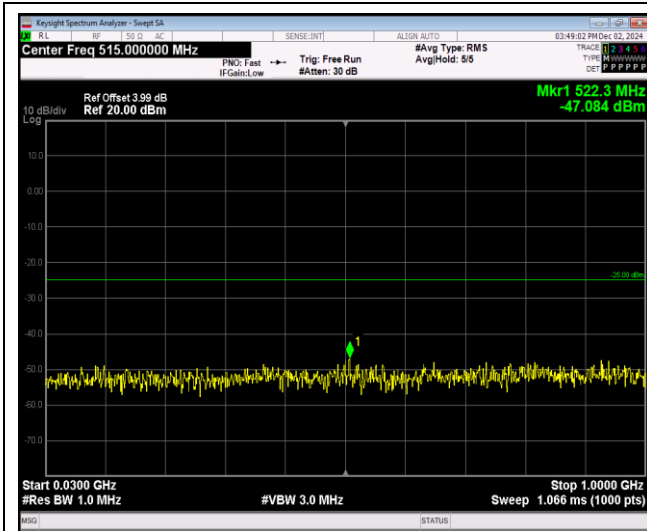
Band41-5MHz-QPSK-41215-1RB#0-Range1:30~100 0MHz
