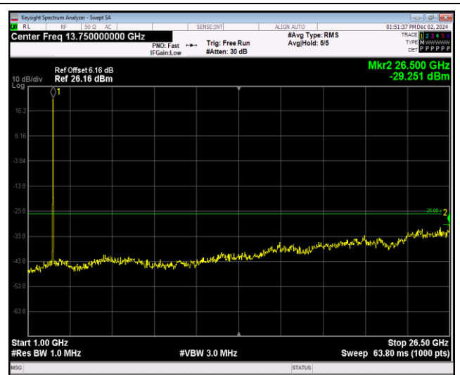
Band7-20MHz-16QAM-21350-1RB#0-Range2:1000~26500MHz
