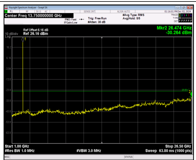
Band7-20MHz-QPSK-20850-1RB#0-Range2:1000~2 6500MHz
