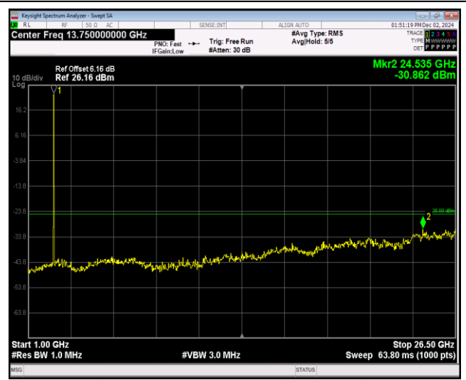
Band7-20MHz-QPSK-21100-1RB#0-Range2:1000~2 6500MHz
