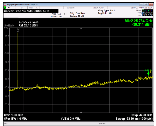
Band7-20MHz-QPSK-21100-1RB#0-Range2:1000~2 6500MHz
