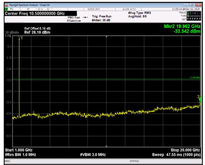
Band4-1.4MHz-QPSK-20175-1RB#0-Range2:1000~20000MHz
