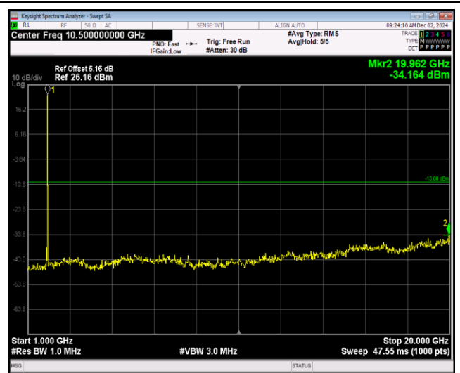
Band4-1.4MHz-QPSK-19957-1RB#0-Range2:1000~20000MHz
