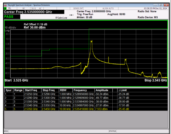
Band41-5MHz-QPSK-40065-25RB#0
