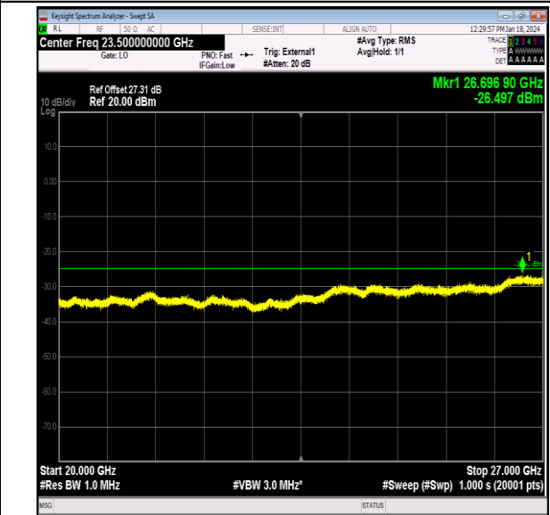
Band41_20MHz_QPSK_40640_1RB#0_20000~27000_20000~27000 000~27000
