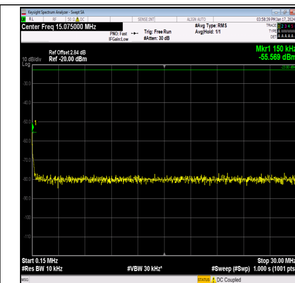
Band26 10MHz QPSK 26915 1RB#0 0.15~30 0.15~30
