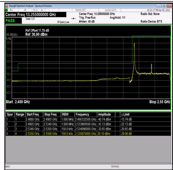
Band41_15MHz_QPSK_40115_1RB#0
