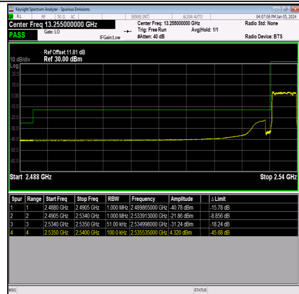
Band41_5MHz_QPSK_40065_25RB#0
