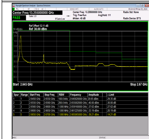
Band41_10MHz_QPSK_41190_1RB#0
