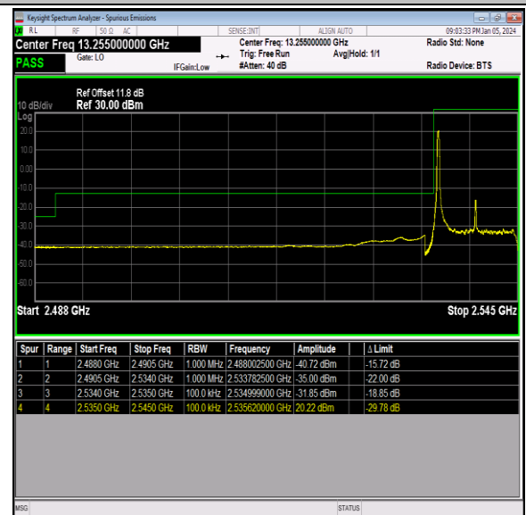
Band41_10MHz_QPSK_40090_1RB#0
