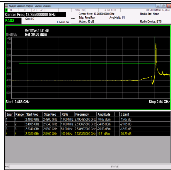
Band41_5MHz_QPSK_40065_1RB#0
