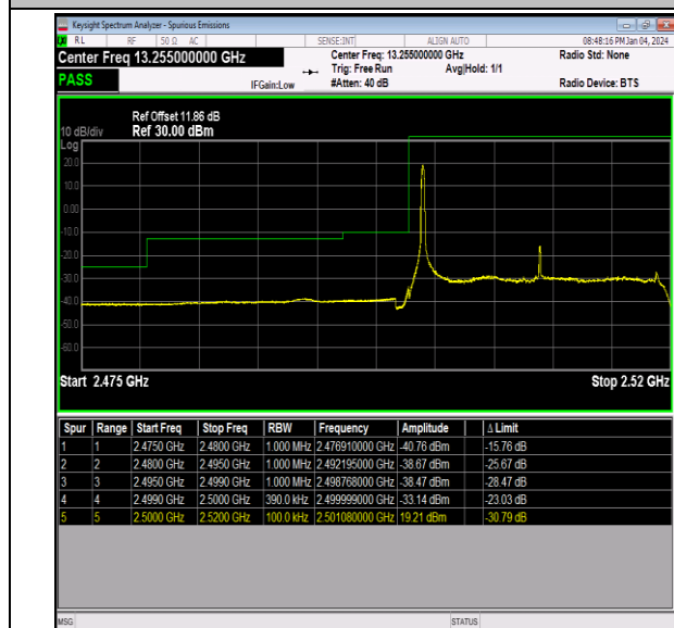
Band7_20MHz_QPSK_20850_1RB#0
