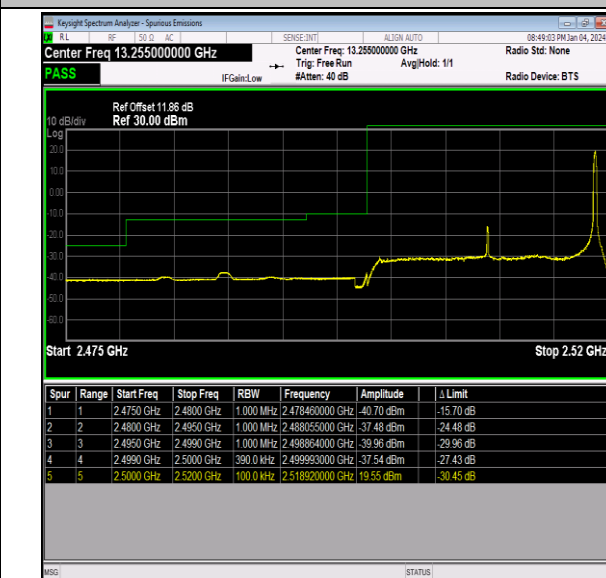
Band7_20MHz_QPSK_20850_1RB#99
