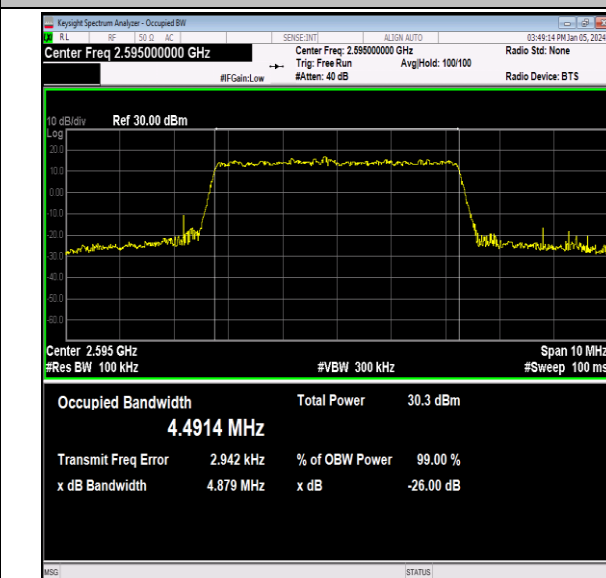
41(2535-2655)-5MHz-16QAM-40640-25RB#0-PASS
