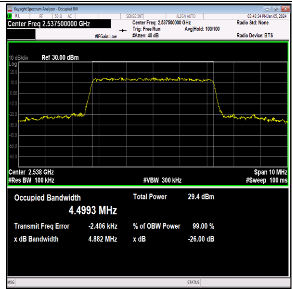
41(2535-2655)-5MHz-64QAM-40065-25RB#0-PASS
