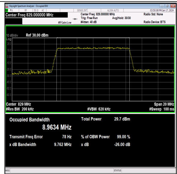
26(824-849)-10MHz-64QAM-26840-50RB#0-PASS
