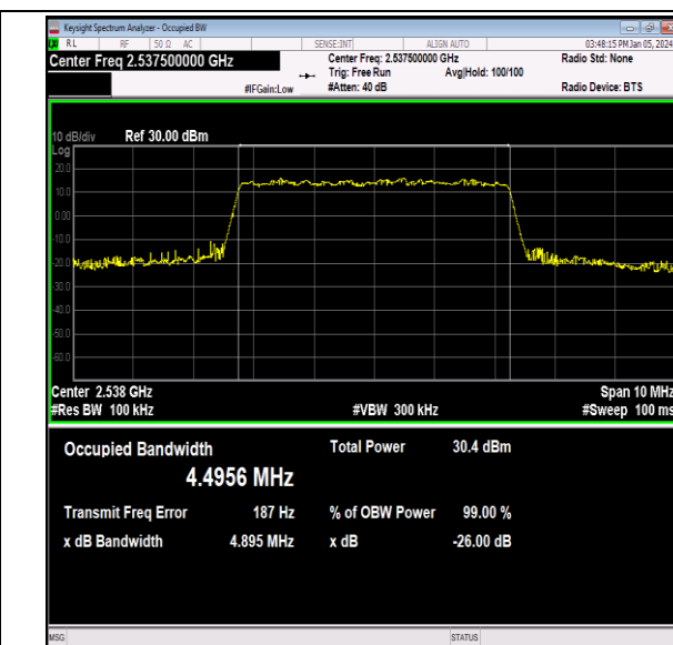
41(2535-2655)-5MHz-16QAM-40065-25RB#0-PASS
