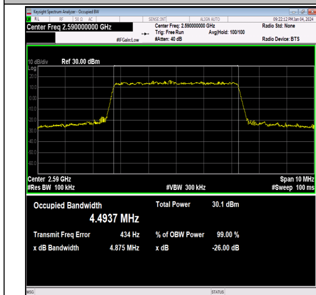
41(2535-2655)-5MHz-16QAM-40590-25RB#0-PASS
