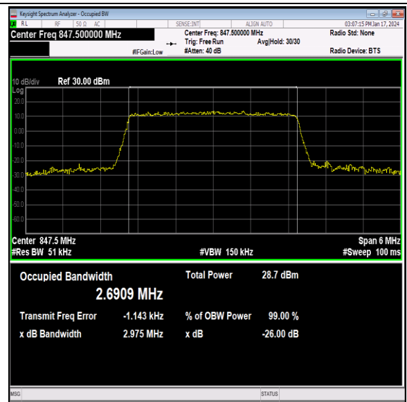
26(824-849)-3MHz-64QAM-27025-15RB#0-PASS
