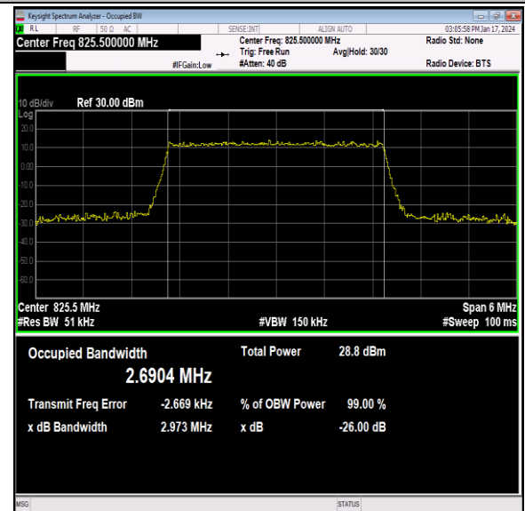
26(824-849)-3MHz-64QAM-26805-15RB#0-PASS
