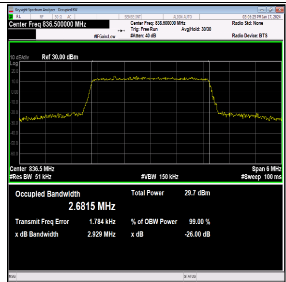
26(824-849)-3MHz-16QAM-26915-15RB#0-PASS
