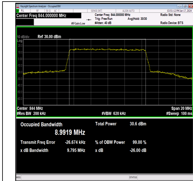
26(824-849)-10MHz-16QAM-26990-50RB#0-PASS
