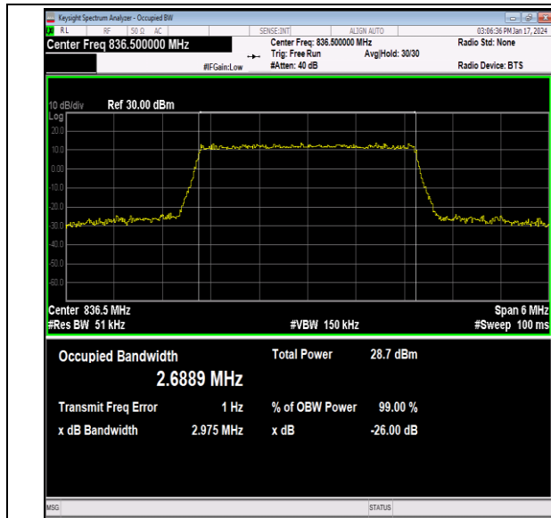
26(824-849)-3MHz-64QAM-26915-15RB#0-PASS
