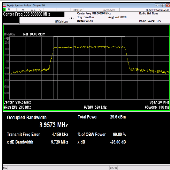
26(824-849)-10MHz-64QAM-26915-50RB#0-PASS
