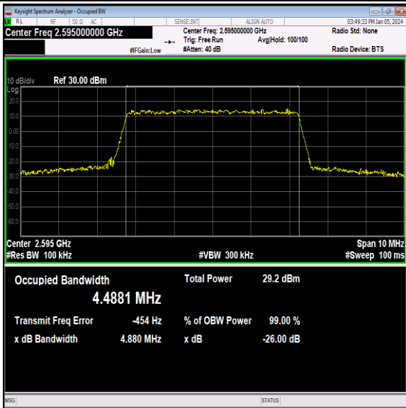
41(2535-2655)-5MHz-64QAM-40640-25RB#0-PASS
