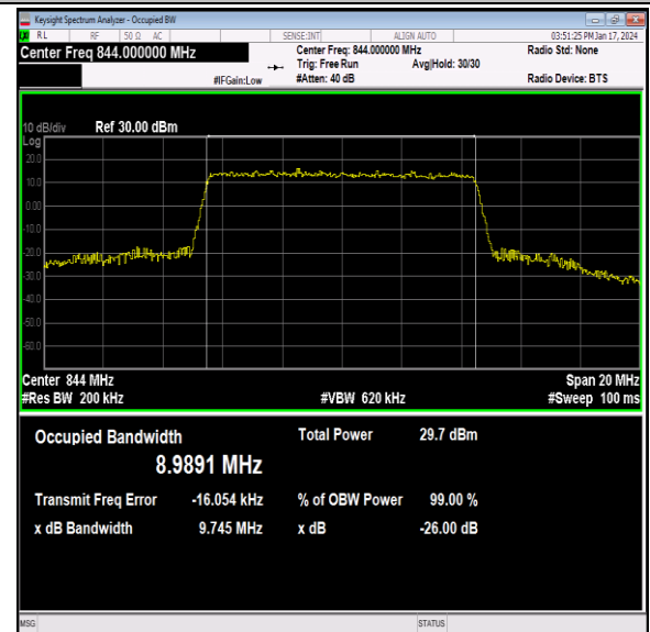
26(824-849)-10MHz-64QAM-26990-50RB#0-PASS
