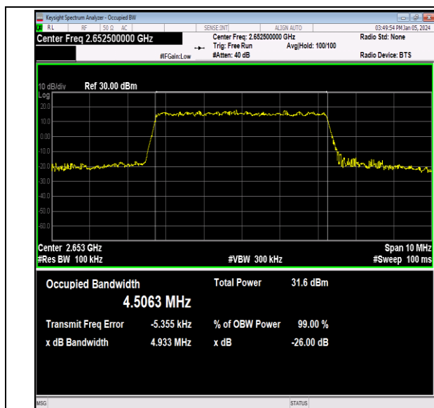
41(2535-2655)-5MHz-QPSK-41215-25RB#0-PASS
