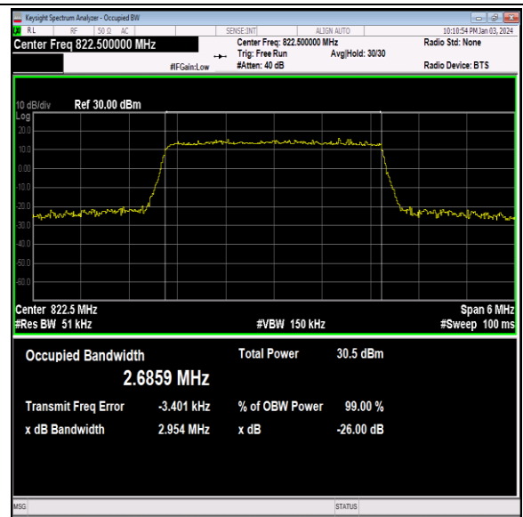
26(814-824)-3MHz-QPSK-26775-15RB#0-PASS
