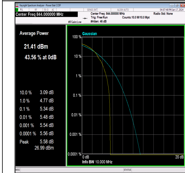
26(824-849)-10MHz-64QAM-26990-1RB#0-PASS
