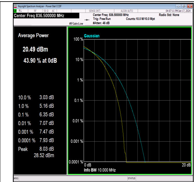
26(824-849)-10MHz-64QAM-26915-50RB#0-PASS
