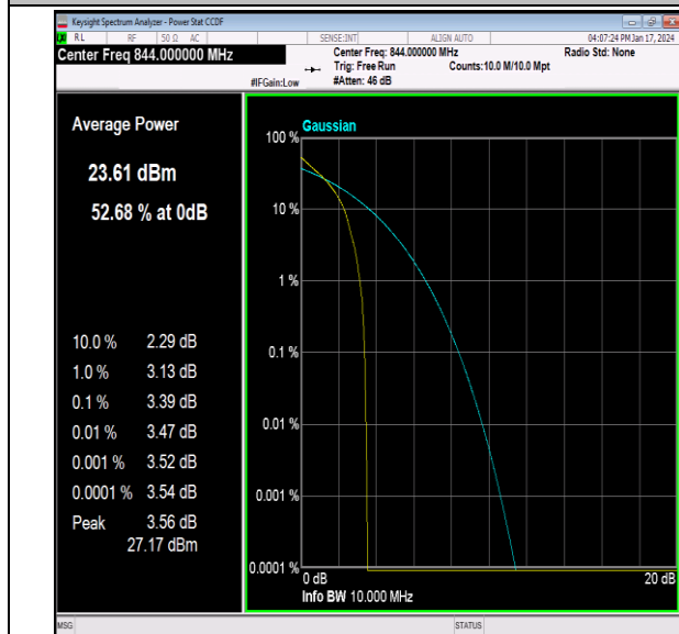
26(824-849)-10MHz-QPSK-26990-1RB#0-PASS
