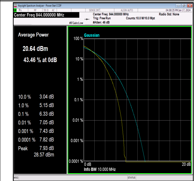
26(824-849)-10MHz-64QAM-26990-50RB#0-PASS
