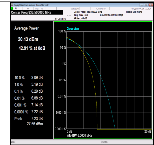
26(824-849)-3MHz-64QAM-26915-15RB#0-PASS
