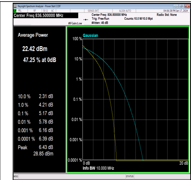
26(824-849)-10MHz-QPSK-26915-50RB#0-PASS
