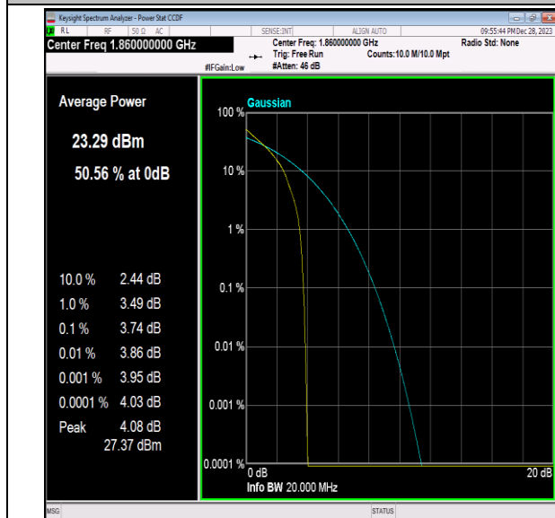
Band2-20MHz-QPSK-18700-1RB#0-PASS
