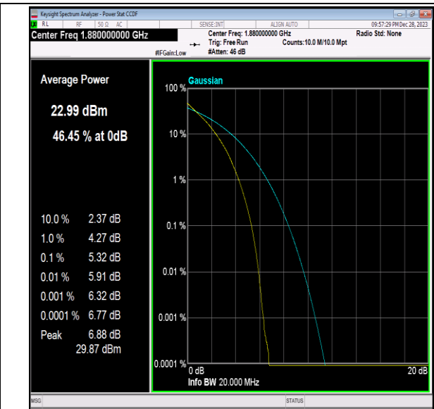
Band2-20MHz-QPSK-18900-100RB#0-PASS
