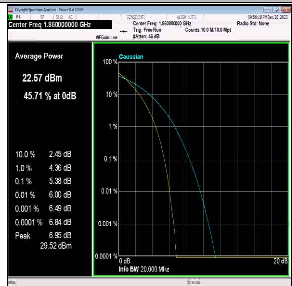
Band2-20MHz-QPSK-18700-100RB#0-PASS
