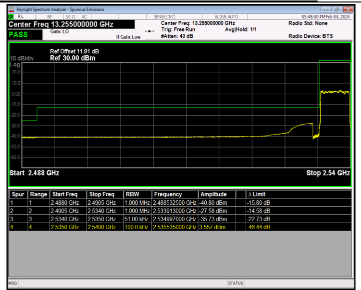
Band41_5MHz_QPSK_40065_25RB#0
