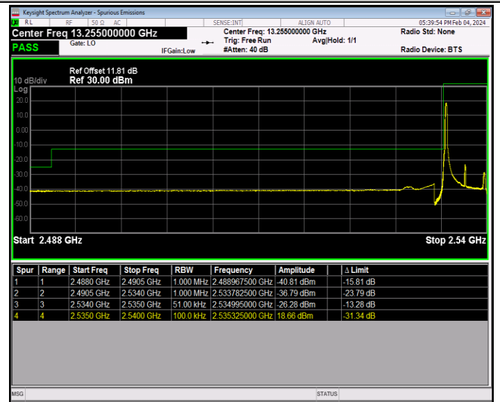
Band41_5MHz_QPSK_40065_1RB#0
