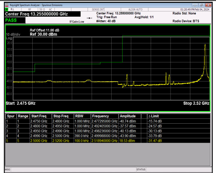
Band7_20MHz_QPSK_20850_1RB#99
