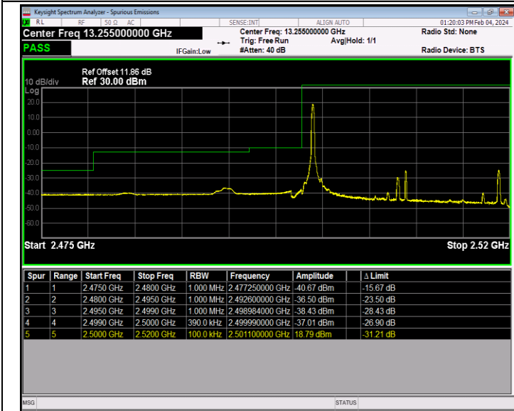
Band7_20MHz_QPSK_20850_1RB#0
