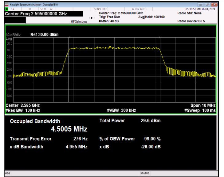
41(2535-2655)-5MHz-16QAM-40640-25RB#0-PASS
