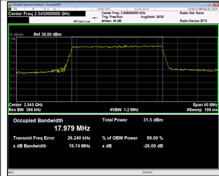
41(2535-2655)-20MHz-QPSK-40140-100RB#0-PASS
