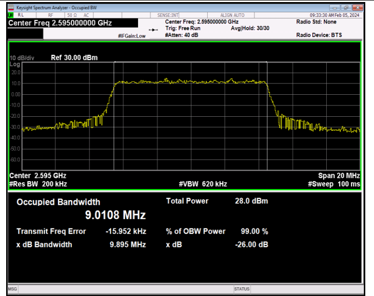
41(2535-2655)-10MHz-64QAM-40640-50RB#0-PASS
