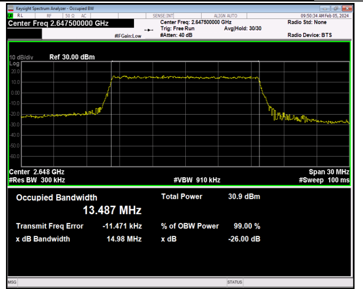
41(2535-2655)-15MHz-QPSK-41165-75RB#0-PASS
