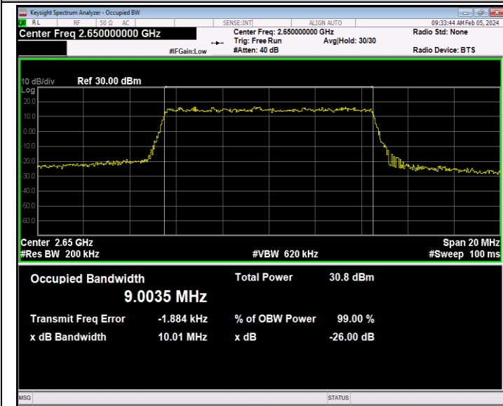
41(2535-2655)-10MHz-QPSK-41190-50RB#0-PASS
