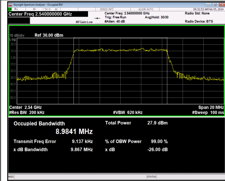
41(2535-2655)-10MHz-64QAM-40090-50RB#0-PASS
