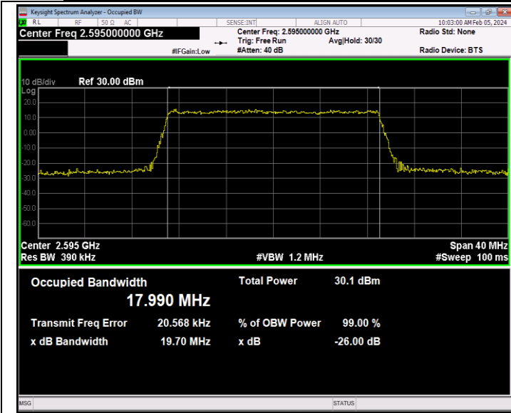
41(2535-2655)-20MHz-16QAM-40640-100RB#0-PASS
