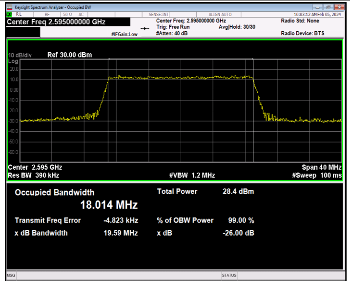
41(2535-2655)-20MHz-64QAM-40640-100RB#0-PASS
