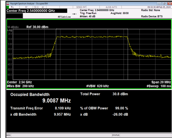
41(2535-2655)-10MHz-QPSK-40090-50RB#0-PASS
