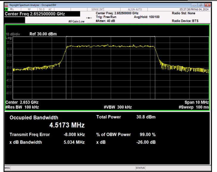
41(2535-2655)-5MHz-QPSK-41215-25RB#0-PASS
