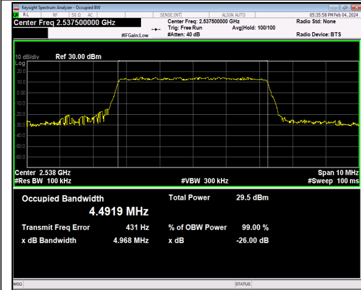
41(2535-2655)-5MHz-16QAM-40065-25RB#0-PASS
