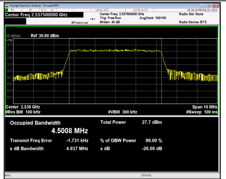
41(2535-2655)-5MHz-64QAM-40065-25RB#0-PASS
