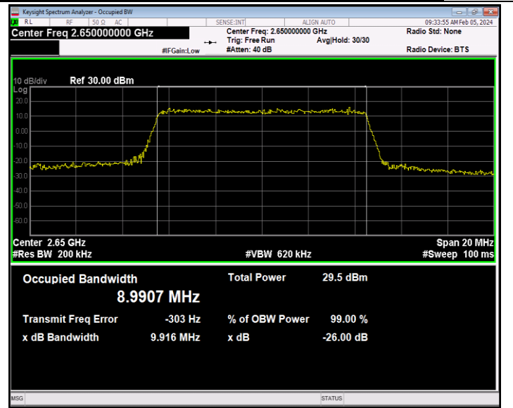
41(2535-2655)-10MHz-16QAM-41190-50RB#0-PASS
