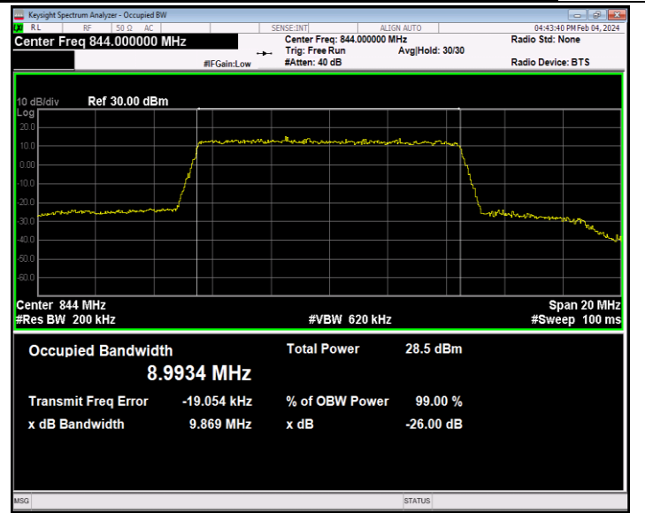
26(824-849)-10MHz-64QAM-26990-50RB#0-PASS
