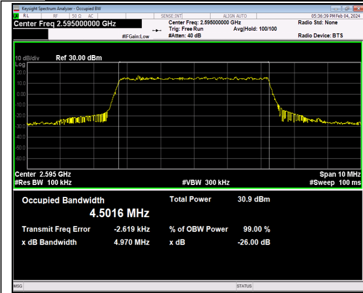
41(2535-2655)-5MHz-QPSK-40640-25RB#0-PASS
