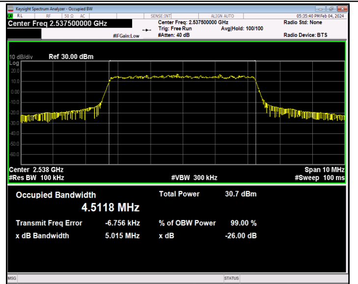
41(2535-2655)-5MHz-QPSK-40065-25RB#0-PASS
