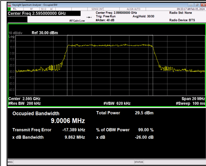
41(2535-2655)-10MHz-16QAM-40640-50RB#0-PASS
