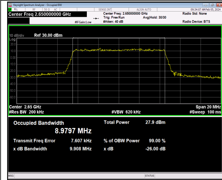
41(2535-2655)-10MHz-64QAM-41190-50RB#0-PASS
