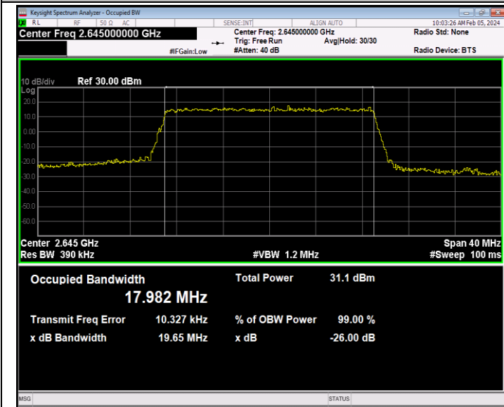
41(2535-2655)-20MHz-QPSK-41140-100RB#0-PASS
