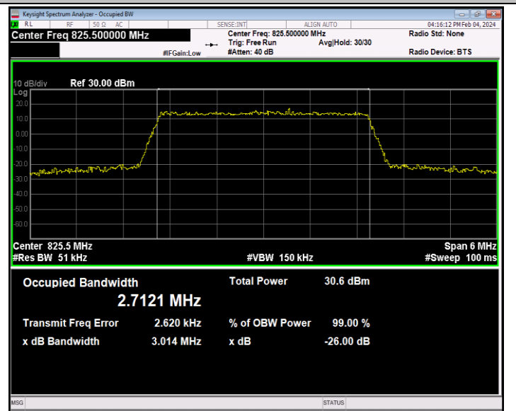
26(824-849)-3MHz-QPSK-26805-15RB#0-PASS
