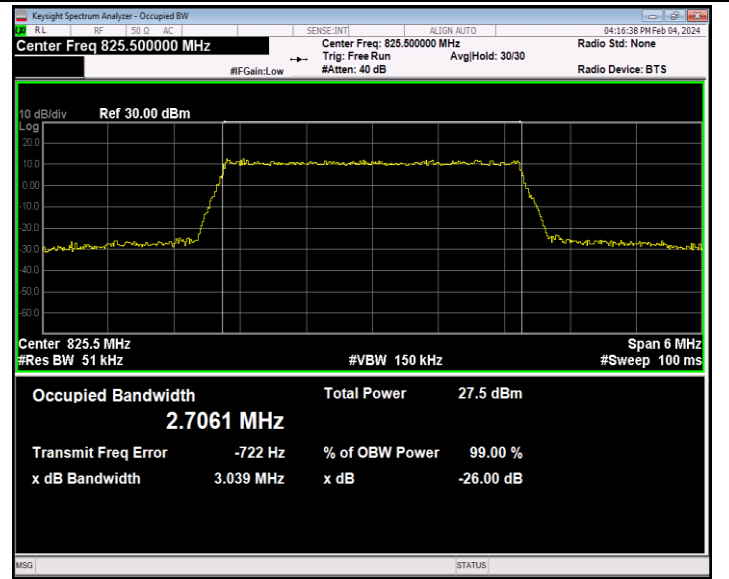
26(824-849)-3MHz-64QAM-26805-15RB#0-PASS
