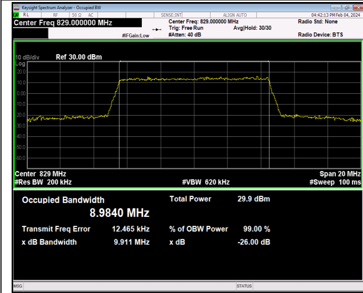
26(824-849)-10MHz-16QAM-26840-50RB#0-PASS
