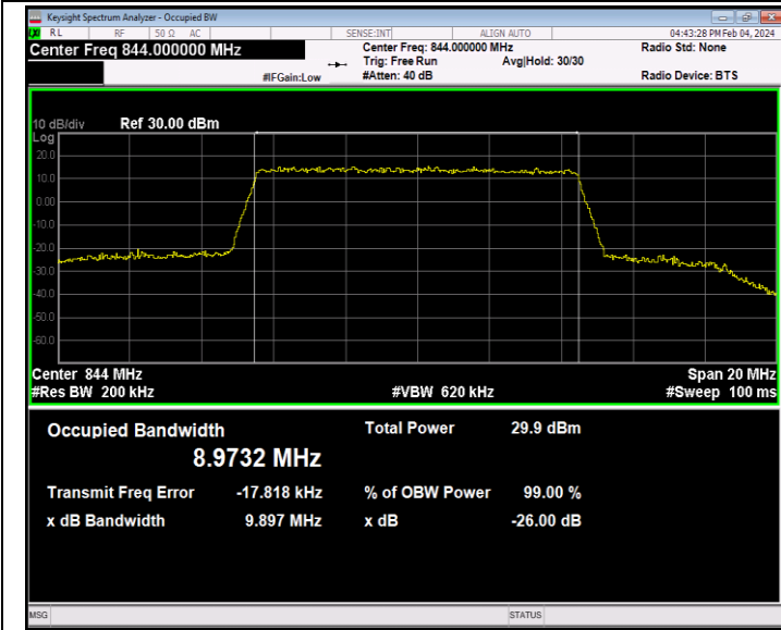
26(824-849)-10MHz-16QAM-26990-50RB#0-PASS
