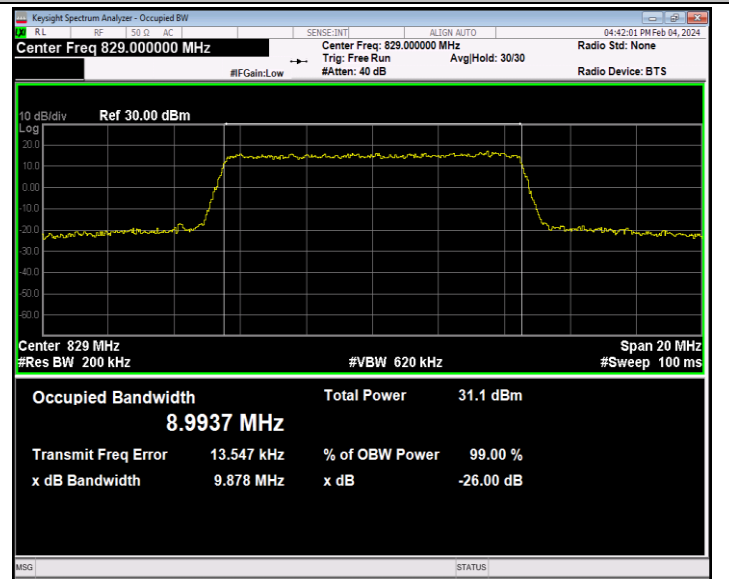
26(824-849)-10MHz-QPSK-26840-50RB#0-PASS
