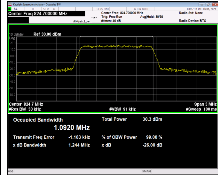
26(824-849)-1.4MHz-QPSK-26797-6RB#0-PASS
