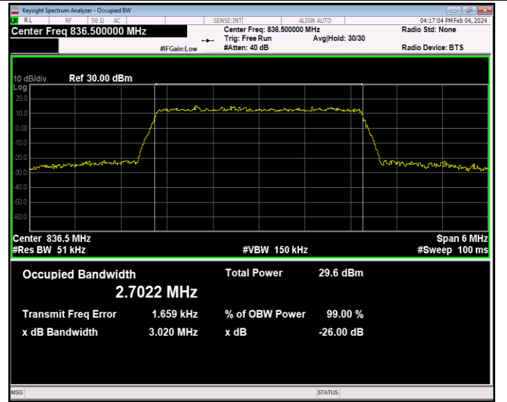
26(824-849)-3MHz-16QAM-26915-15RB#0-PASS
