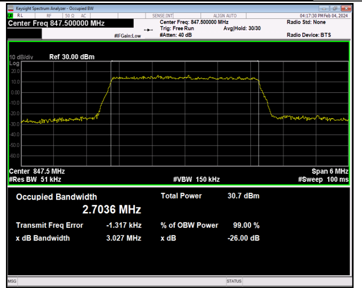
26(824-849)-3MHz-QPSK-27025-15RB#0-PASS
