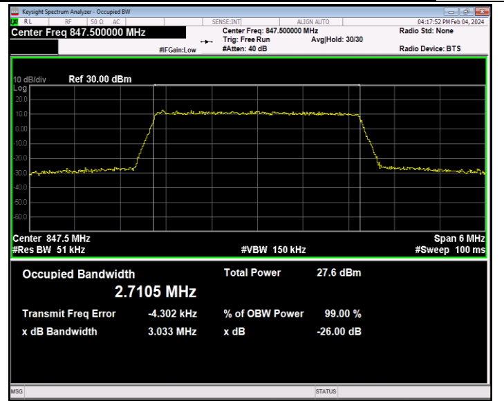
26(824-849)-3MHz-64QAM-27025-15RB#0-PASS
