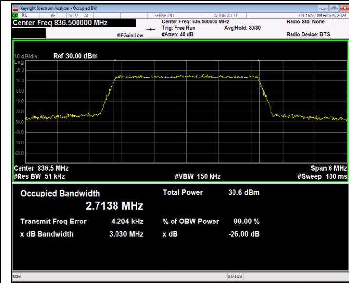
26(824-849)-3MHz-QPSK-26915-15RB#0-PASS
