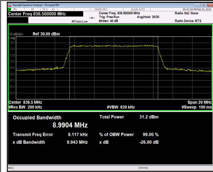
26(824-849)-10MHz-QPSK-26915-50RB#0-PASS
