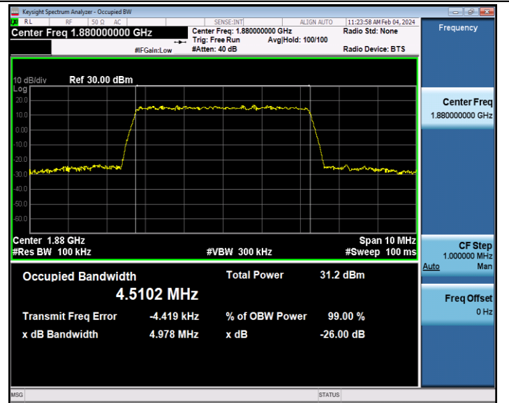
Band2-5MHz-QPSK-18900-25RB#0-PASS
