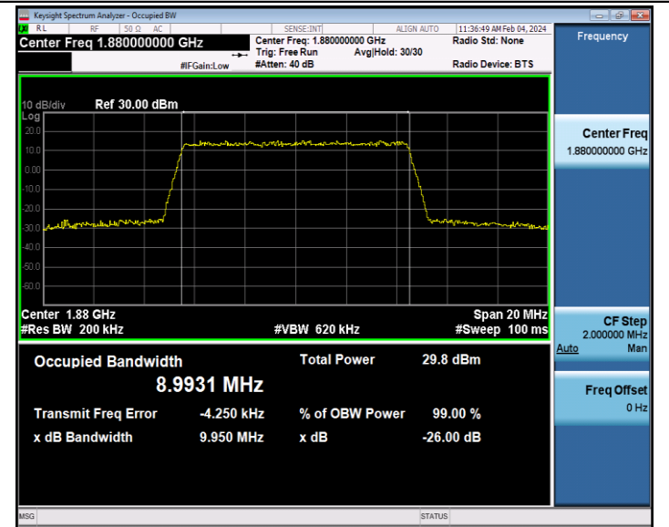
Band2-10MHz-QPSK-18800-50RB#0-PASS
