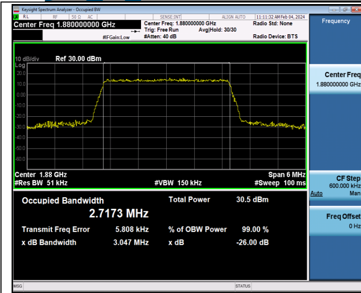
Band2-3MHz-QPSK-18900-15RB#0-PASS
