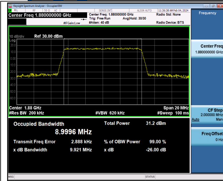
Band2-10MHz-QPSK-18900-50RB#0-PASS
