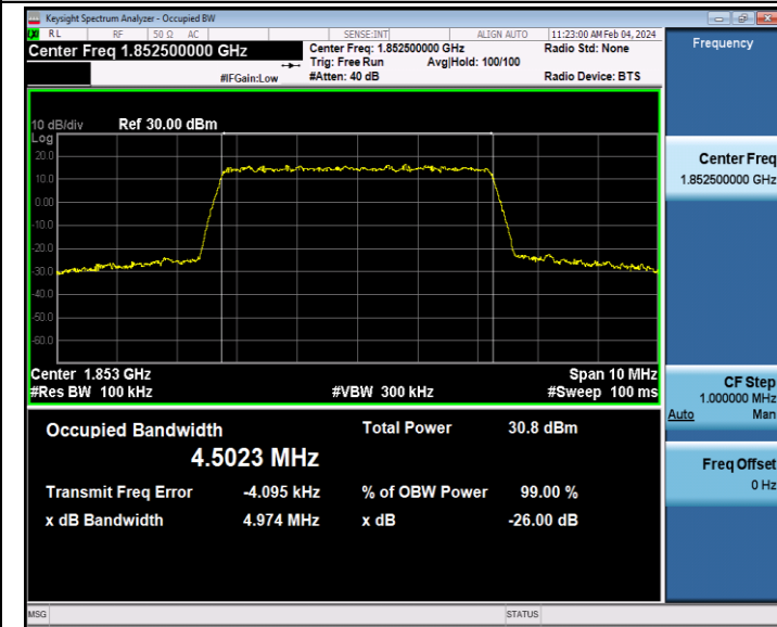
Band2-5MHz-QPSK-18625-25RB#0-PASS
