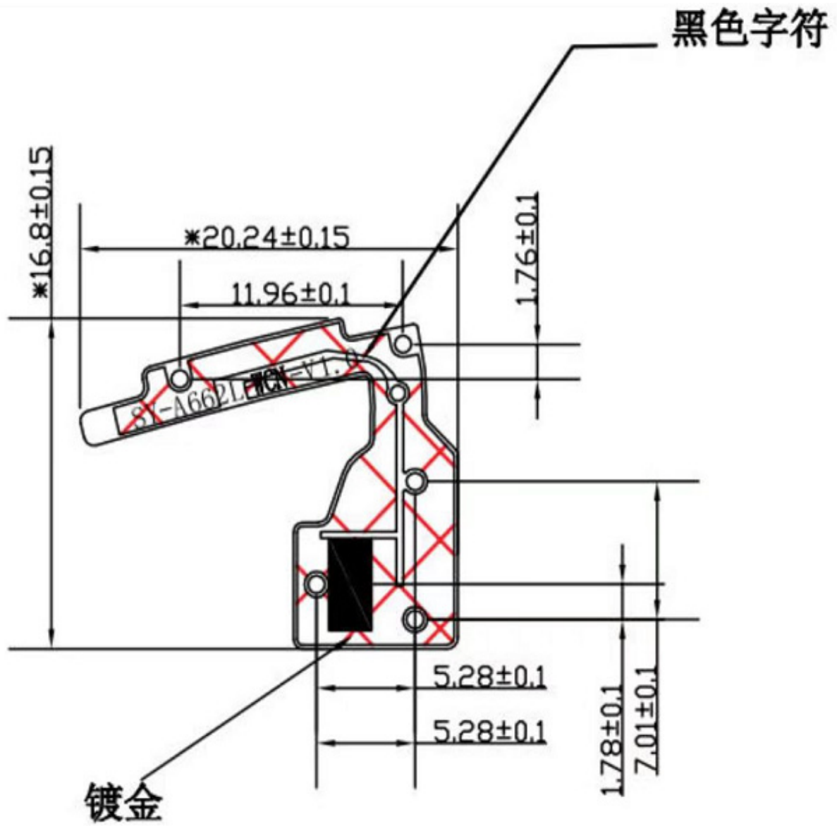
SY-A662L-WCN-V1.0
