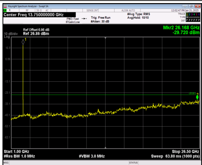
Band38-20MHz-QPSK-37850-1RB#0-Range2:1000~26500MHz
