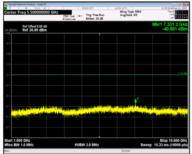
Band26-1.4MHz-QPSK-26797-1RB#0-Range2:1000~10000MHz
