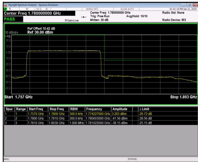
Band66-20MHz-16QAM-132072-1RB#99
