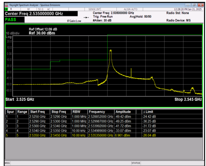
Band41-5MHz-QPSK-40065-25RB#0
