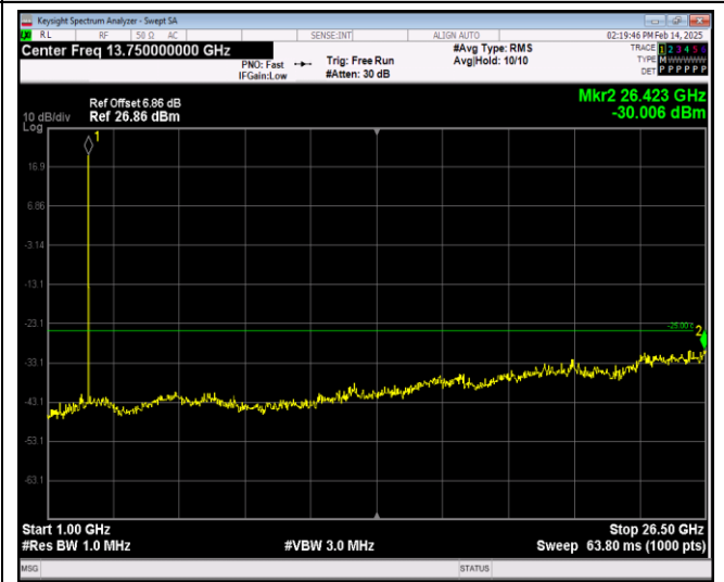
Band38-5MHz-QPSK-38000-1RB#0-Range2:1000~2 6500MHz
