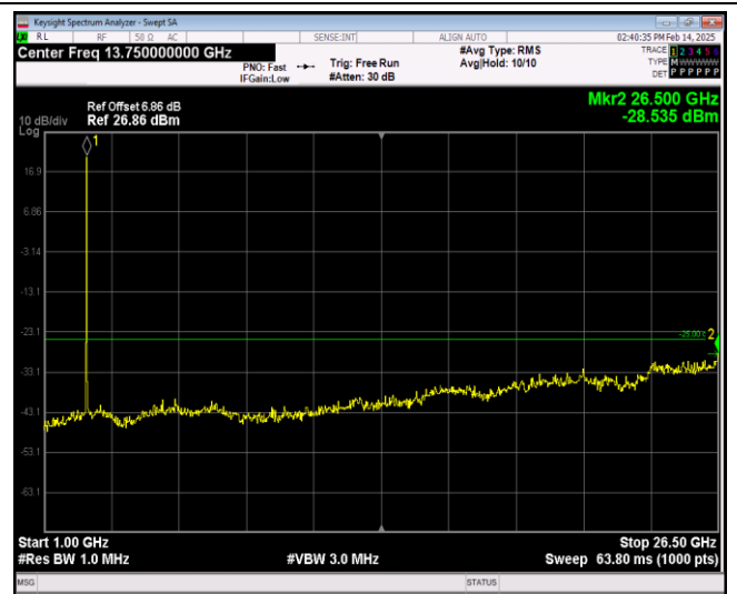
Band38-20MHz-64QAM-37850-1RB#0-Range2:1000~26500MHz
