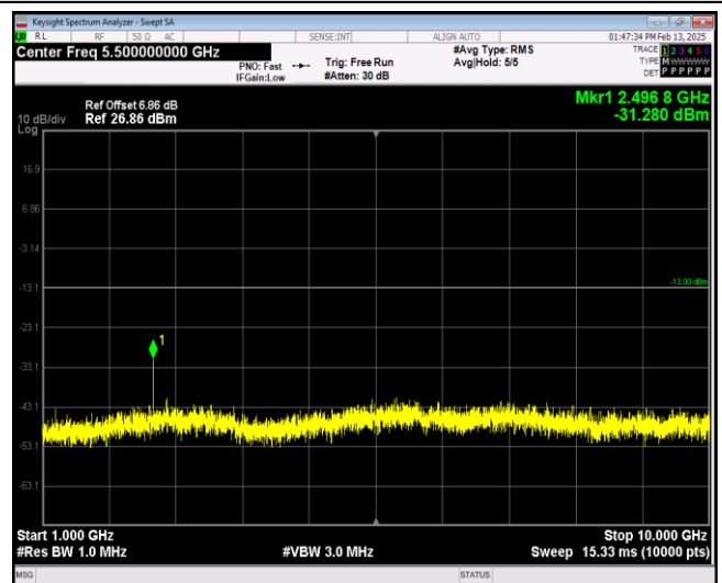
Band5-10MHz-QPSK-20600-1RB#0-Range2:1000~1 0000MHz
