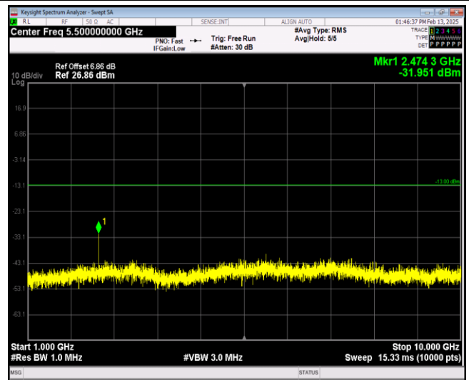
Band5-10MHz-QPSK-20525-1RB#0-Range2:1000~1 0000MHz
