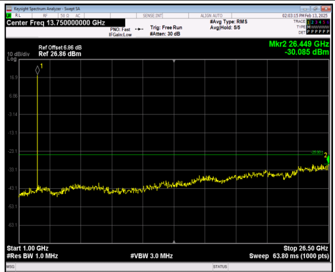
Band7-5MHz-QPSK-21425-1RB#0-Range2:1000~26 500MHz
