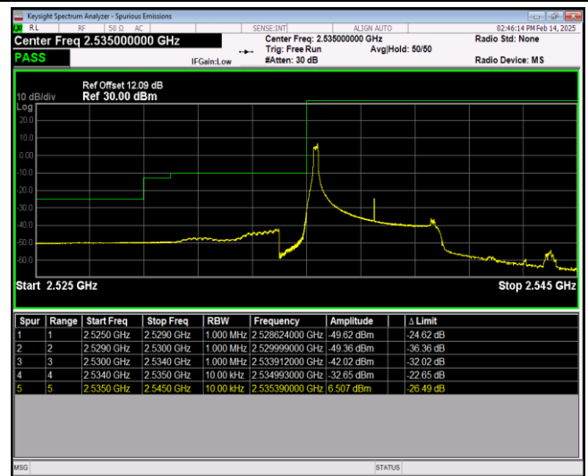
Band41-5MHz-QPSK-40065-25RB#0
