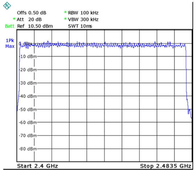
Modulation: \pi/4 DQPSK
