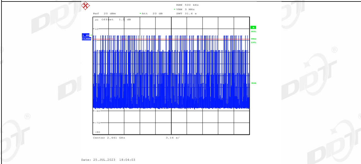
3DH1_Ant1_Hop
