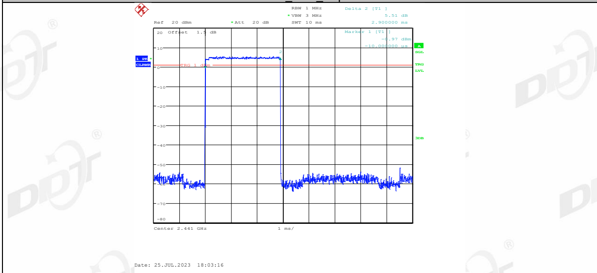
2DH5_Ant1_Hop
