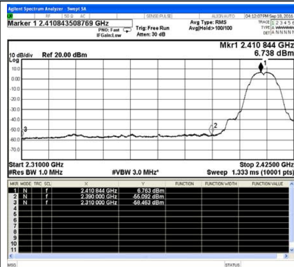
802.11b-Low channel(Average)
