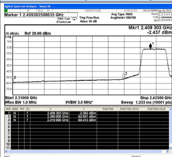
802.11g-Low channel(Average)
