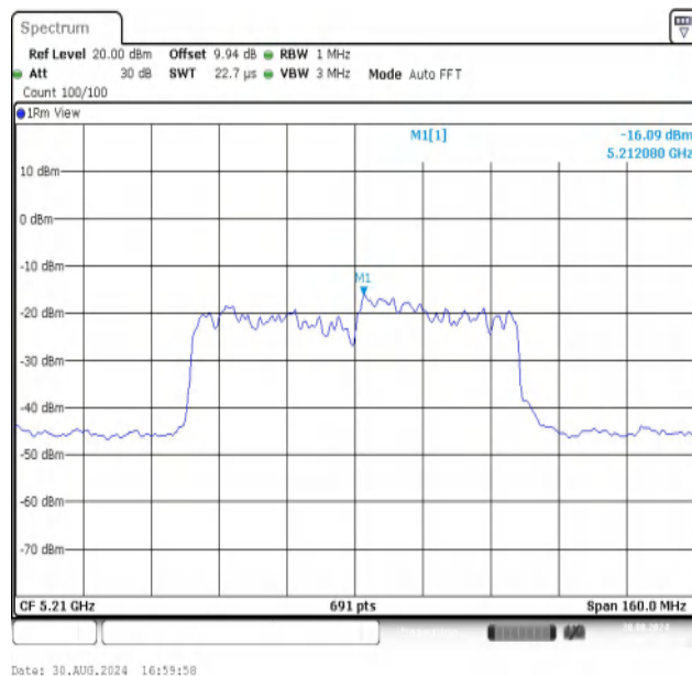
11AC80SISO-Ant1-5210-PASS
