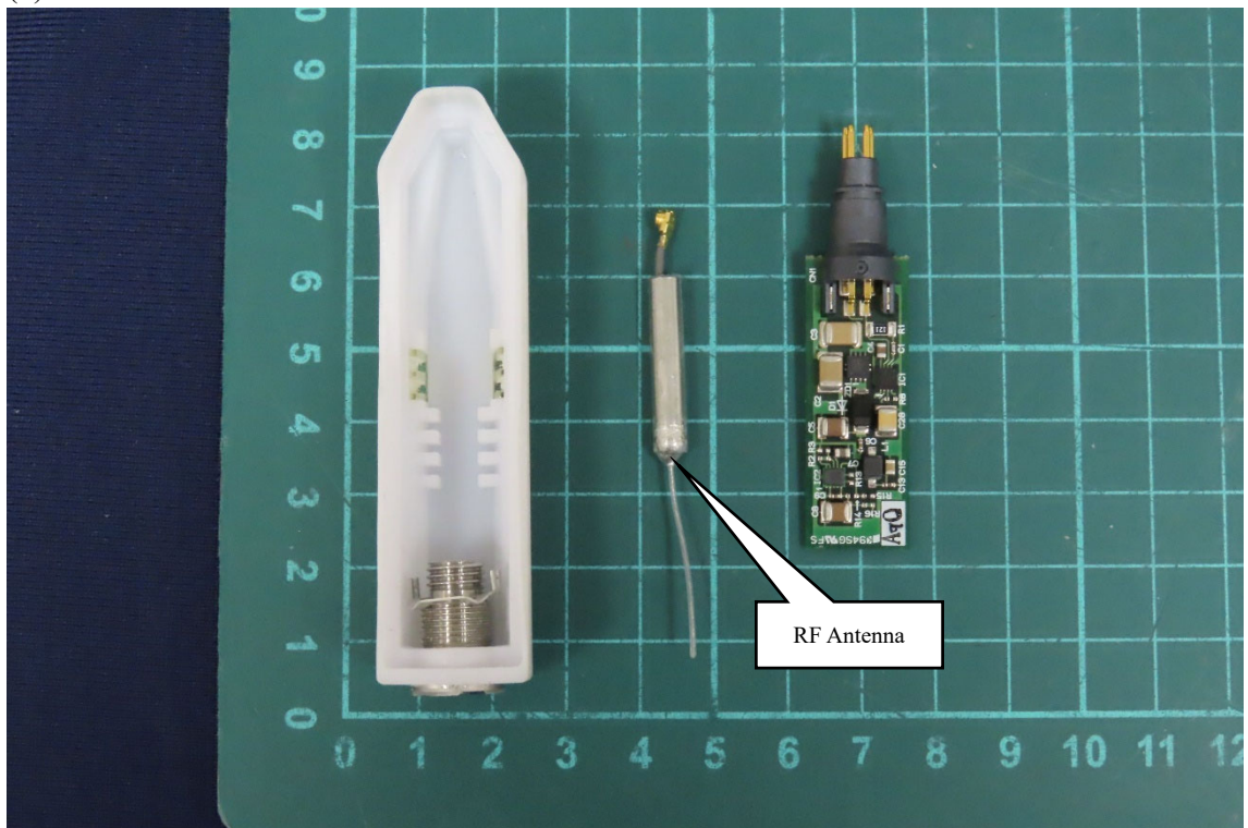
(3) EUT Photo
