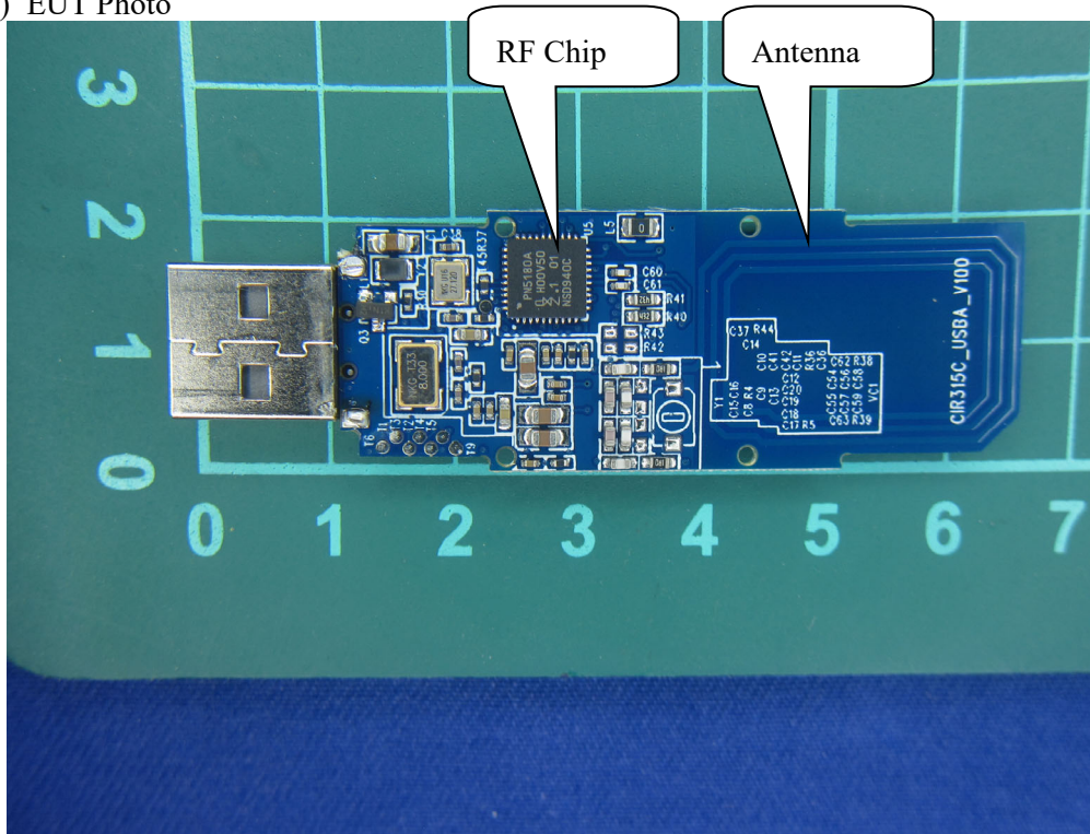
(12) EUT Photo
