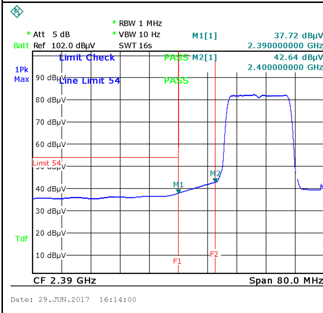
Band Edge, Left Side (Average) - 802.11g Note: F1 is frequency 2390MHz;
