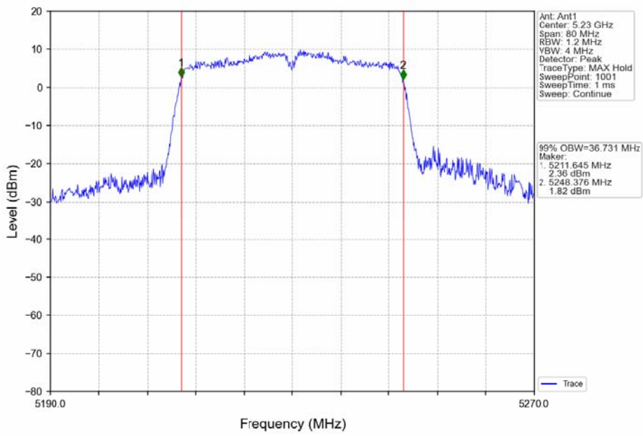
802.11n(HT40)_HCH_5230MHz_Ant1_NTNV
