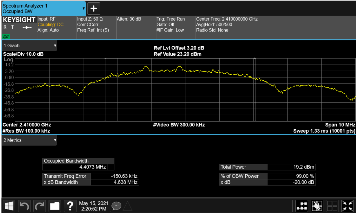
OBW NVNT SRD 2410MHz Ant1
