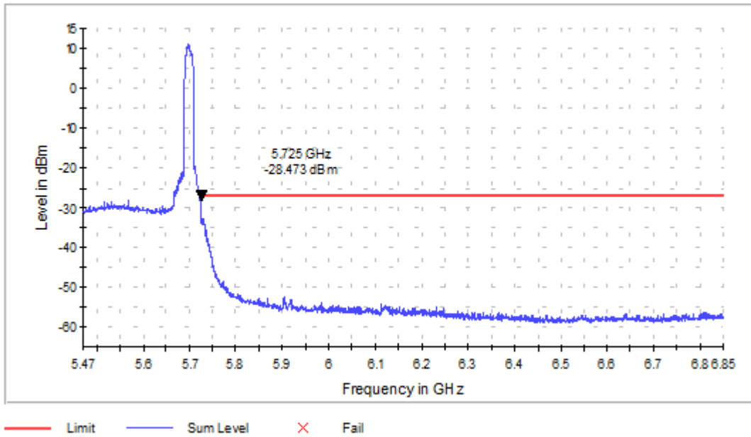
Band Edge
