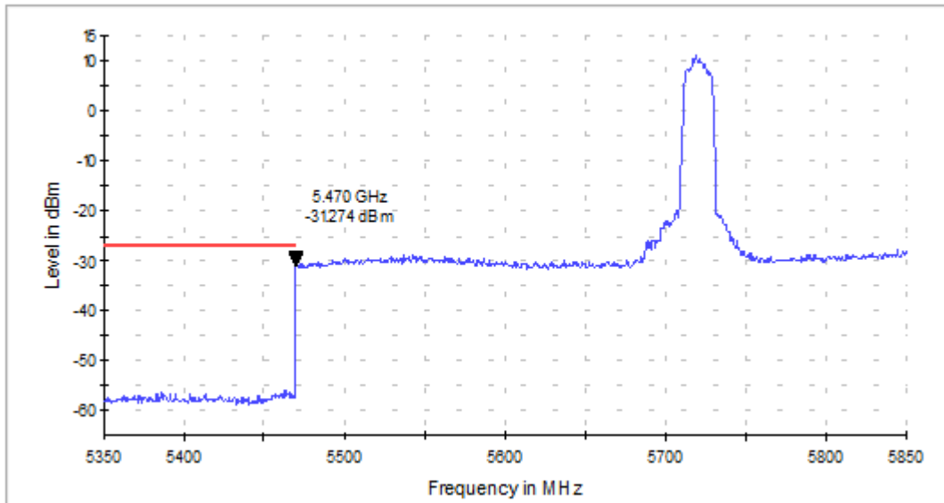
Band Edge
