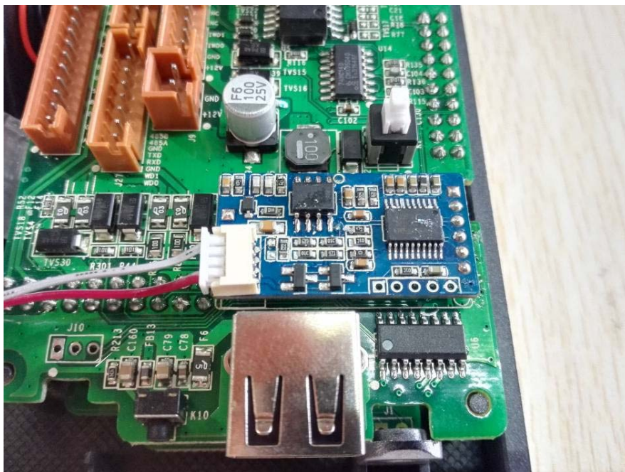
125KHz Module
