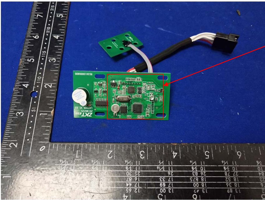
RFID Module
