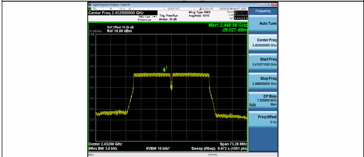
11N40SISO Ant1 2452
