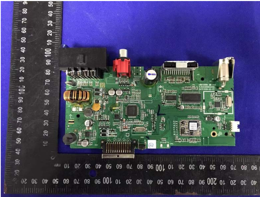
Internal photos M/N:Colombo ML110 BT
