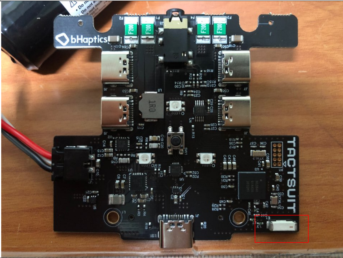
ANTENNA(2.4 GHz)
