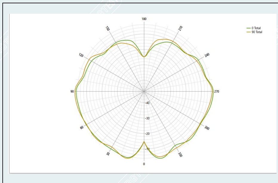
Phi=0 &amp; Phi=90 °_2400MHz
