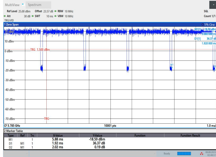
11N20SISO_Ant2_5785
