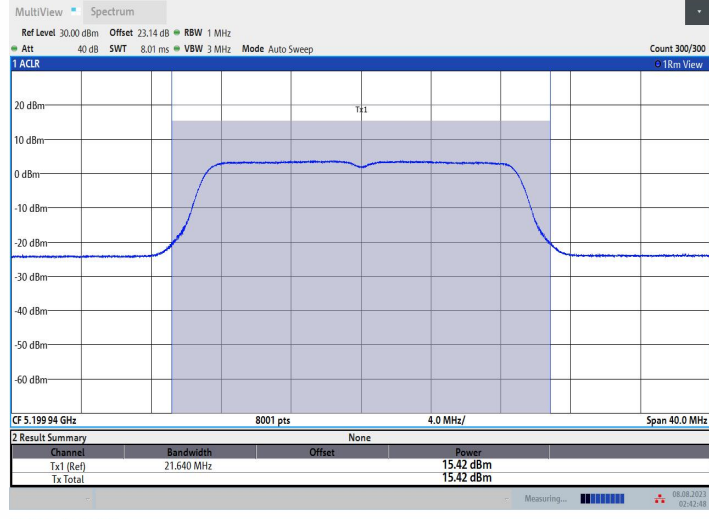
11N20SISO_Ant2_5200
