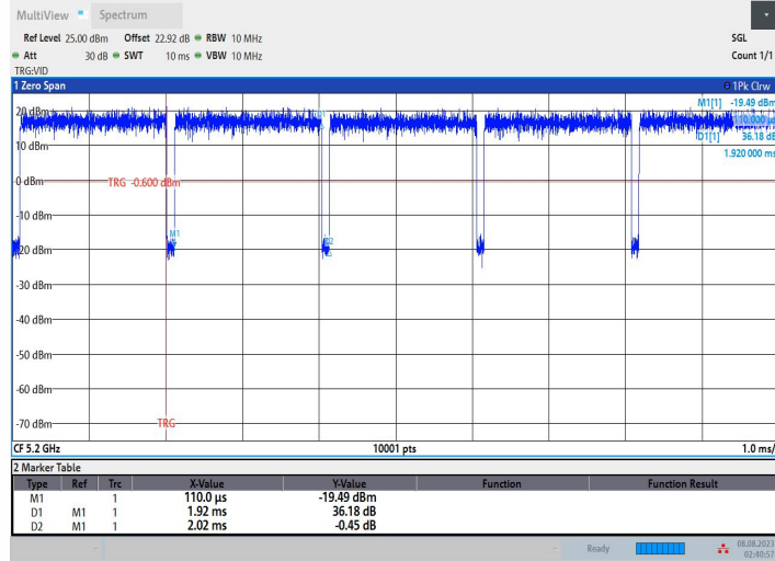
11N20SISO_Ant2_5200
