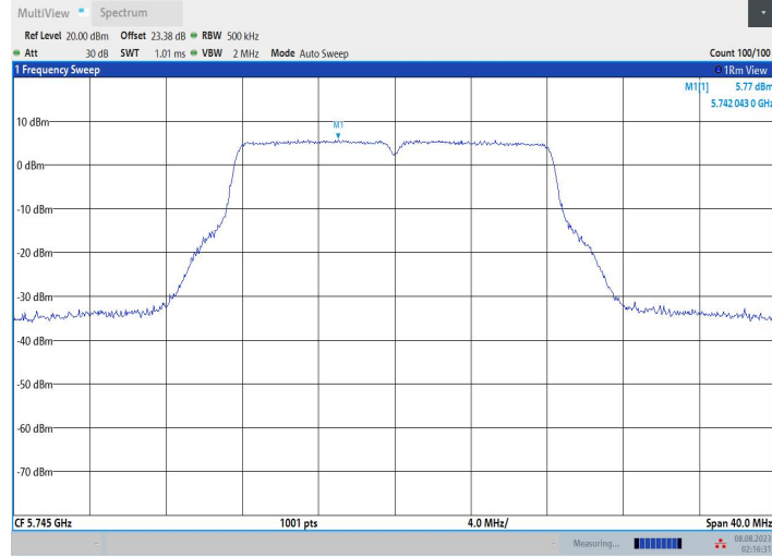
11A_Ant2_5745
