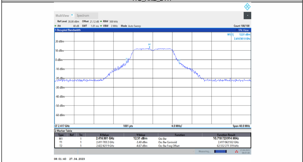
11N20SISO_Ant1_2417
