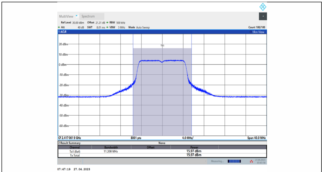
11N20SISO_Ant2_2417
