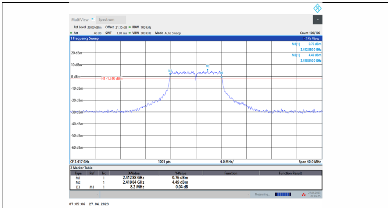
11G_Ant2_2417
