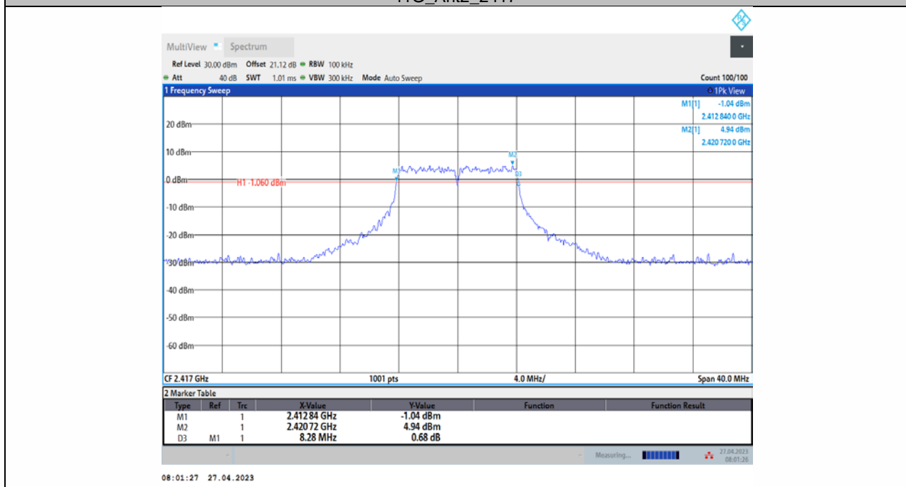
11N20SISO_Ant1_2417
