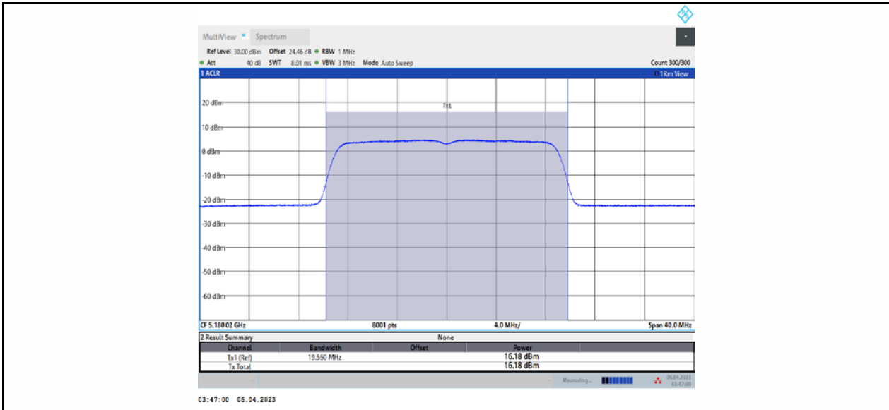
11N20MIMO_Ant2_5180
