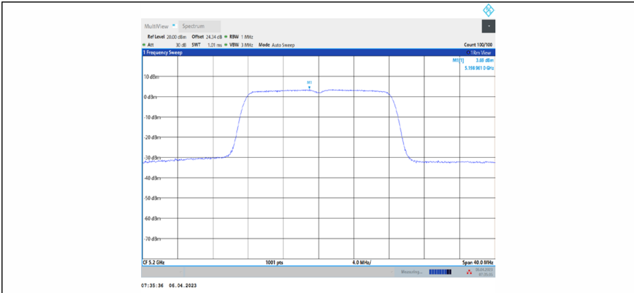
11A_Ant2_5200
