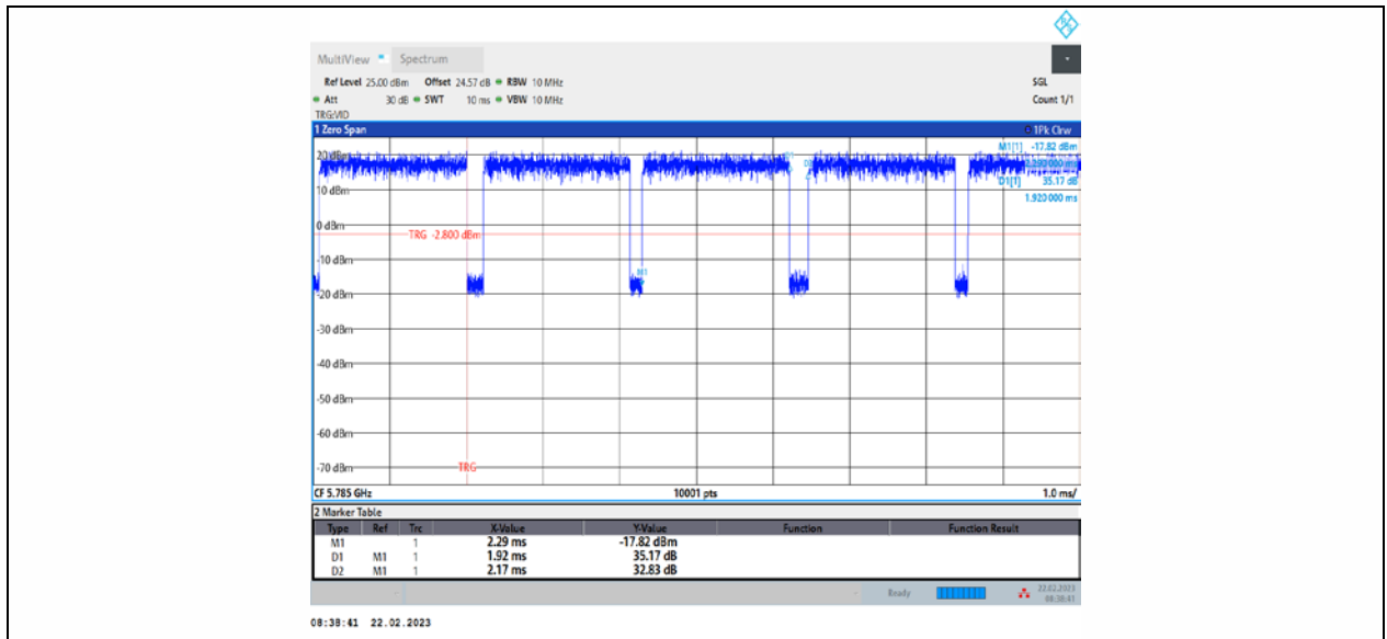
11N20MIMO_Ant2_5785
