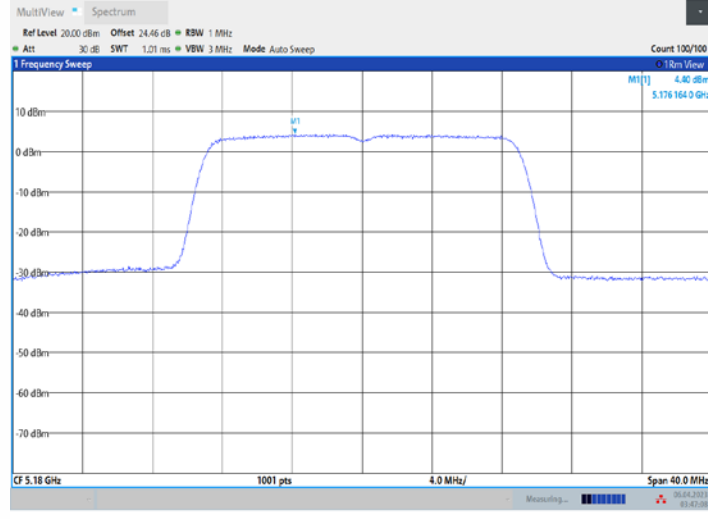
11N20MIMO_Ant2_5180
