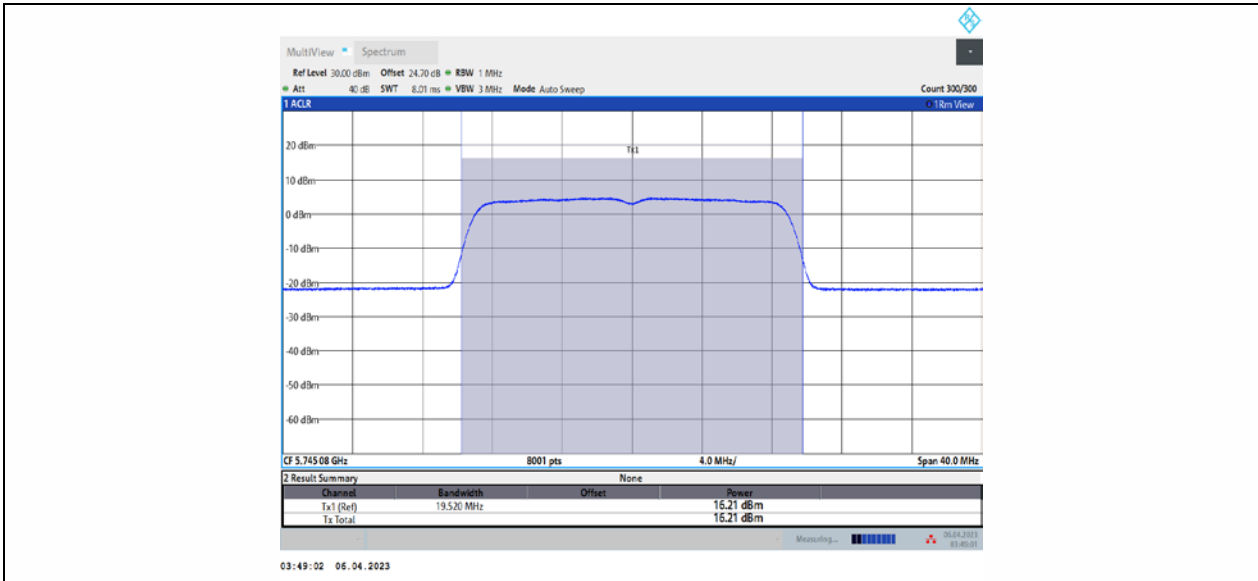
11N20MIMO_Ant2_5745
