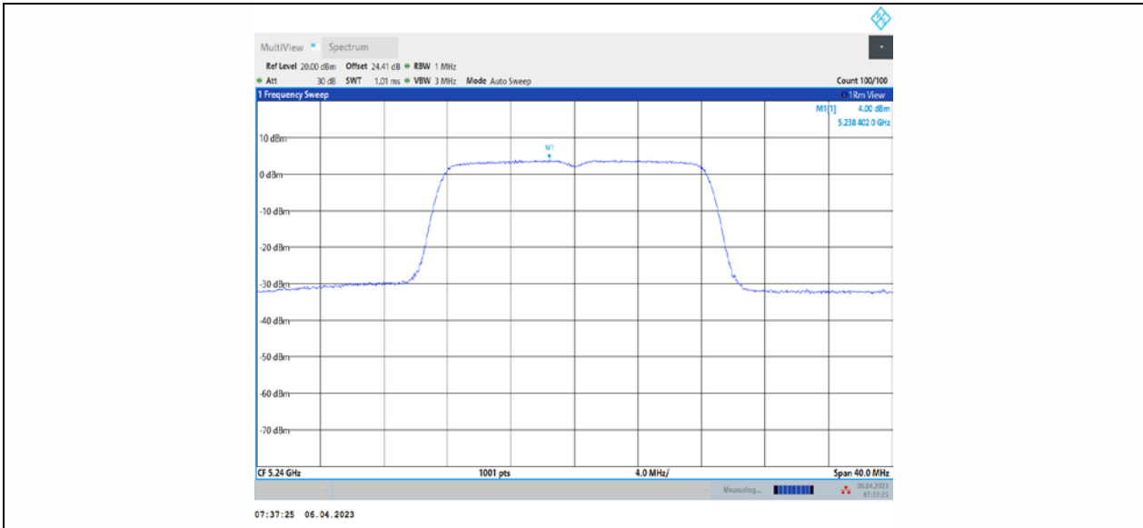
11A_Ant2_5240
