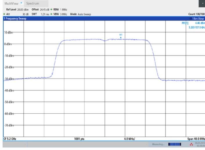
11N20MIMO_Ant2_5200
