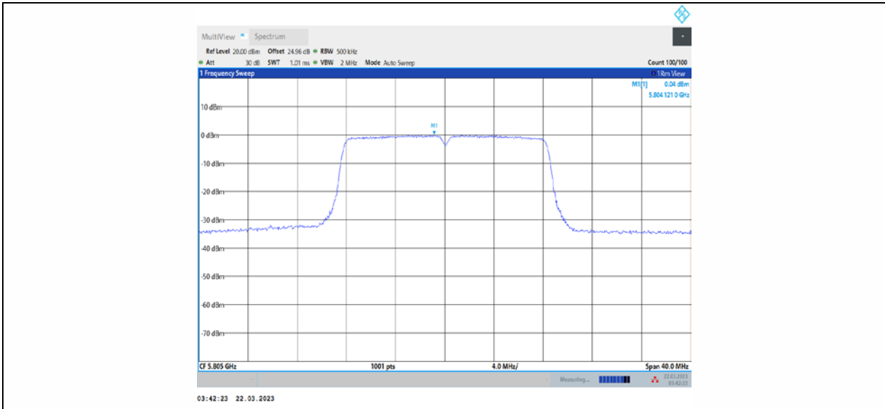
11A_Ant2_5805
