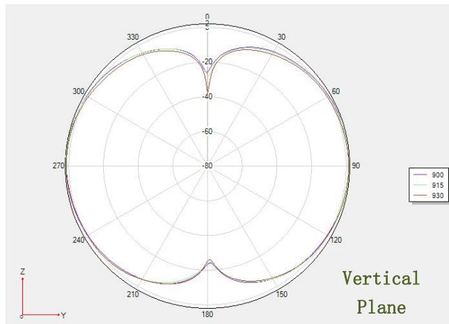
Phi 90 2D 图
