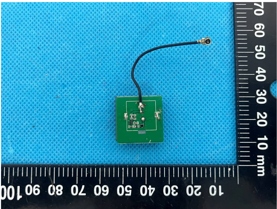
GPS Antenna
