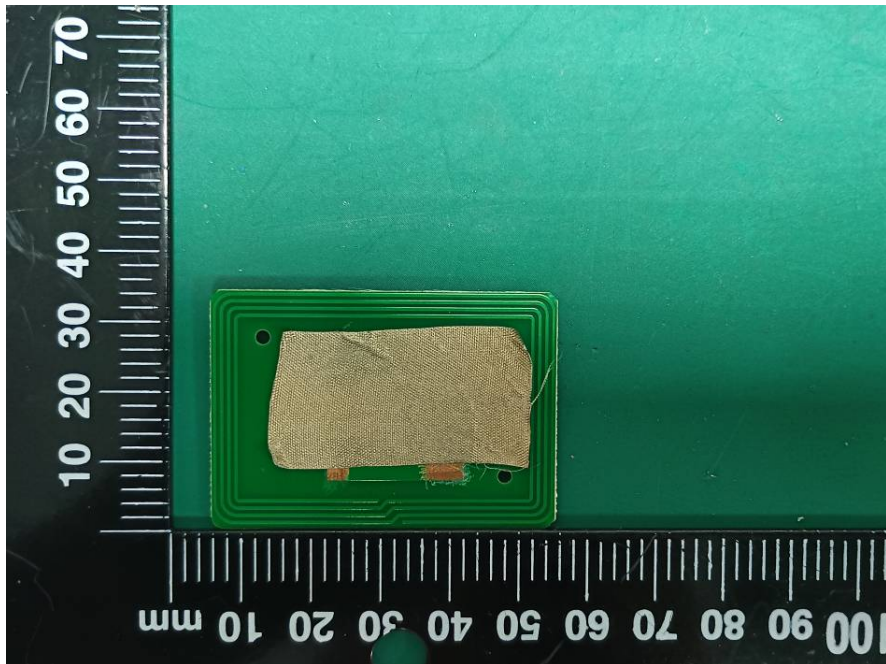
NFC Antenna
